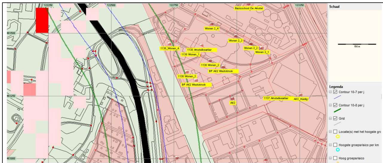
Figuur 25: Plaatsgebonden risicocontouren weg, de groene en blauwe contouren, er zijn uitsluitend een PR 10^{-7} en 10^{-8} contour.
