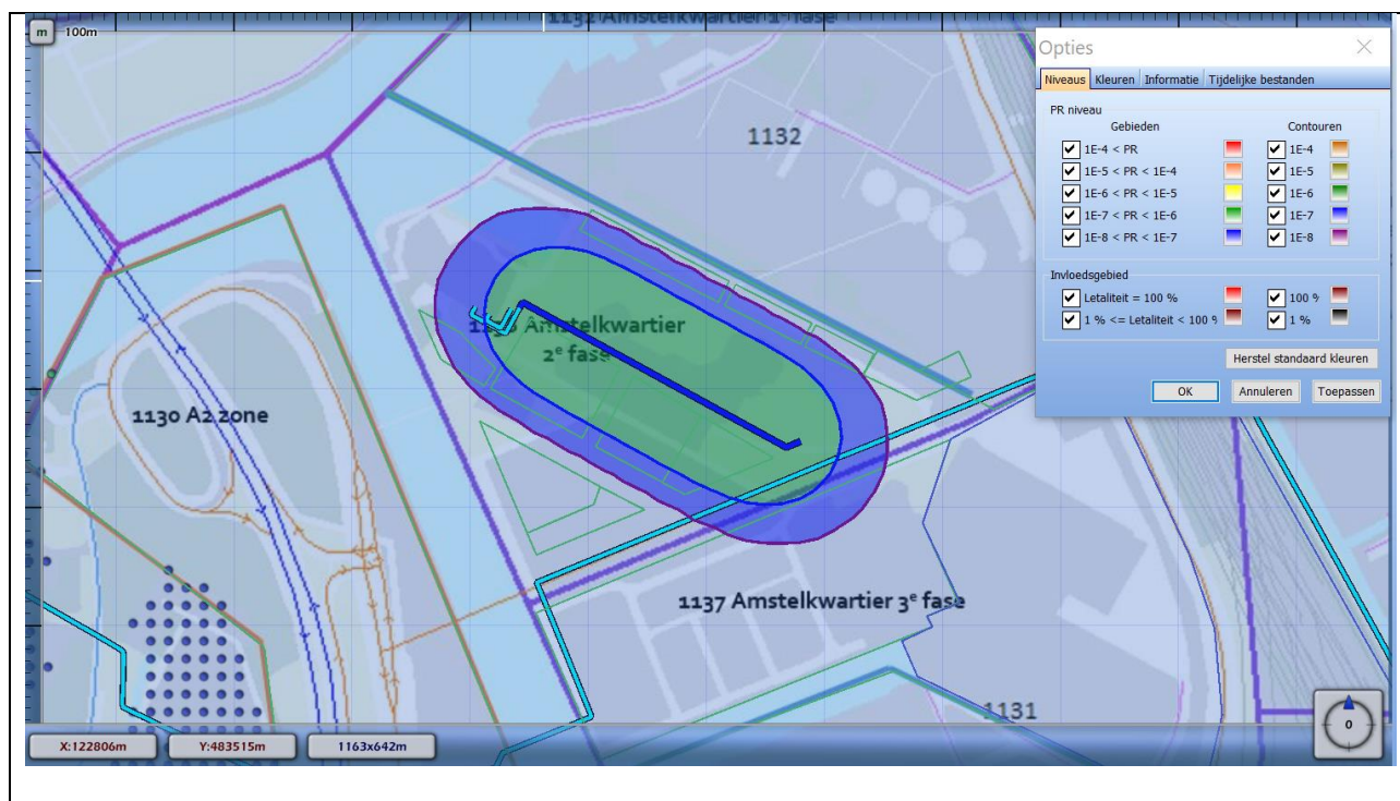
Figuur 8: Weergave van het plaatsgebonden risico voor de leiding 3869_leiding-W-534-02-deel-1.
