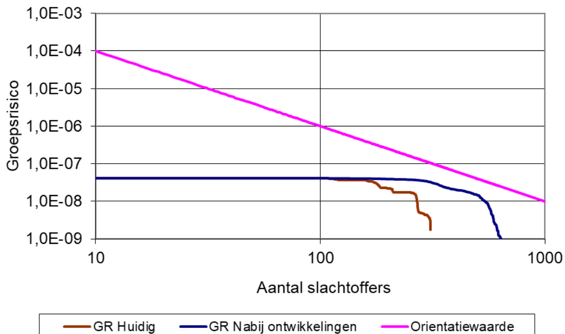
Figuur 18: Groepsrisicocurve bij het plangebied, huidige en toekomstige situatie, 3869_leiding-W-534-XX-deel-1, stationing 20.
