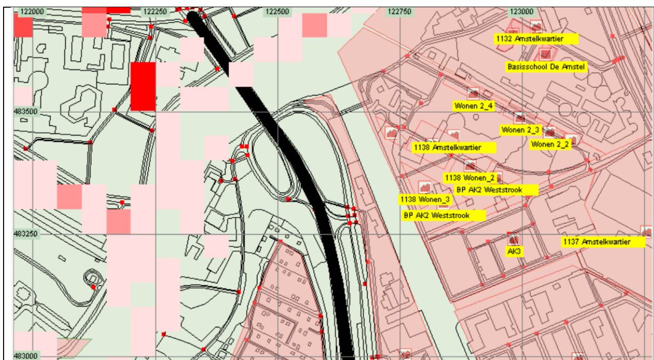
Figuur 5: Ligging van de transportroute weg (A2) nabij het plangebied. Het invloedsgebied van de route over de weg bedraagt 355 m (brandbaar gas). De ruimtelijke ontwikkelingen liggen hier binnen.
