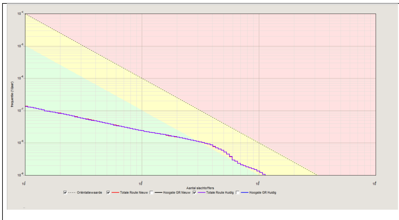
Figuur 23: Groepsrisicocurve spoor, hoogste groepsrisico per kilometer, huidige en nieuwe situatie.
