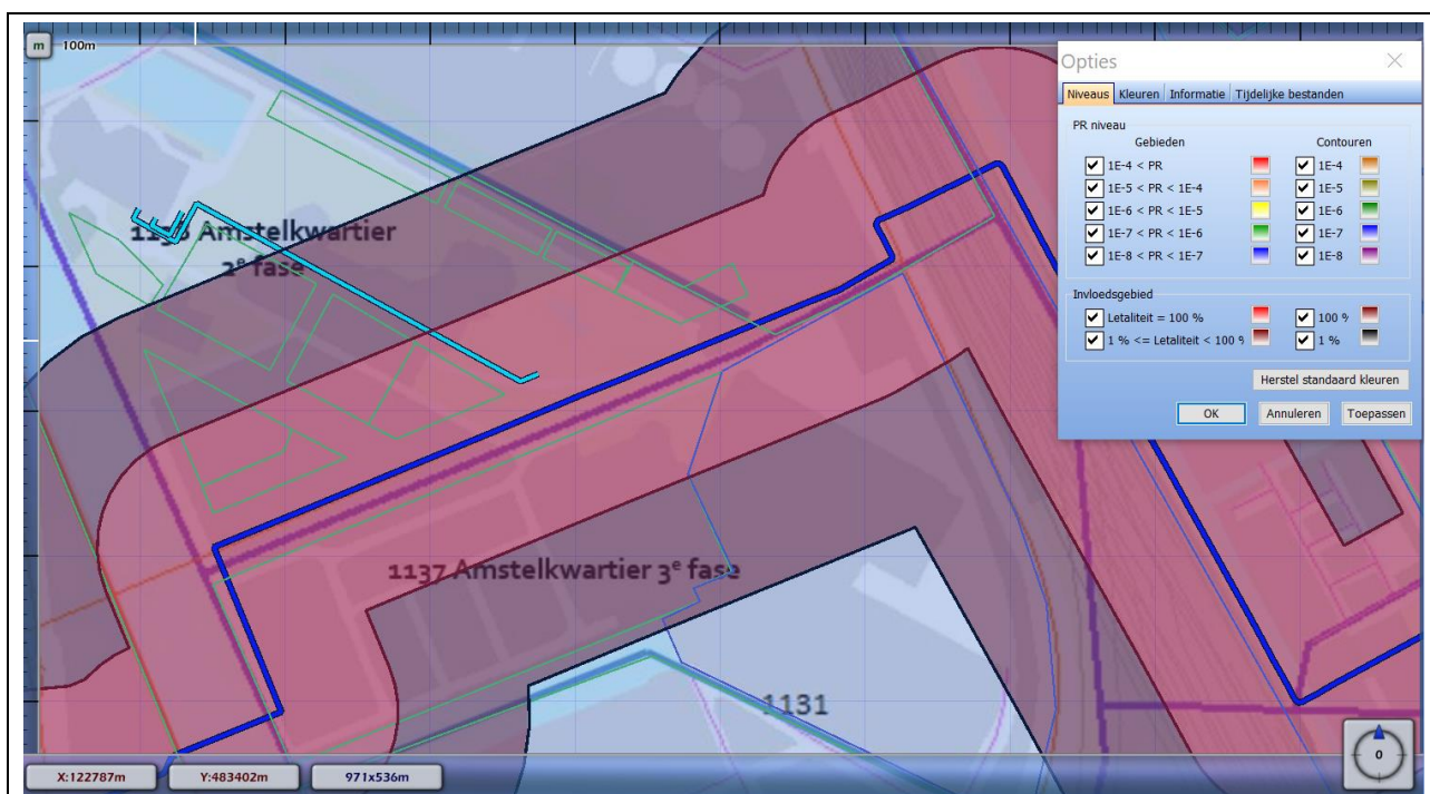
Figuur 13: Invloedsgebied van het groepsrisico voor de 4371_leiding-W-534-01-deel-1_incl verl.
