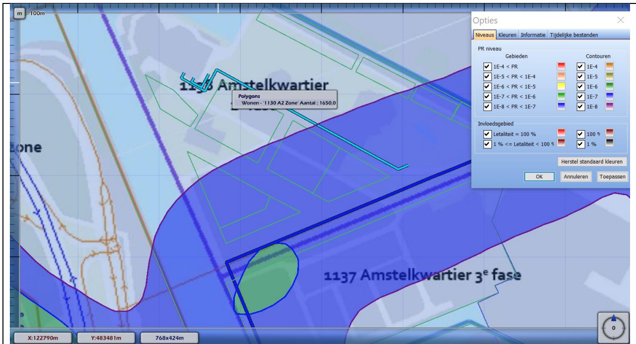
Figuur 10: Weergave van het plaatsgebonden risico voor de 4371_leiding-W-534-01-deel-1_incl verl.
