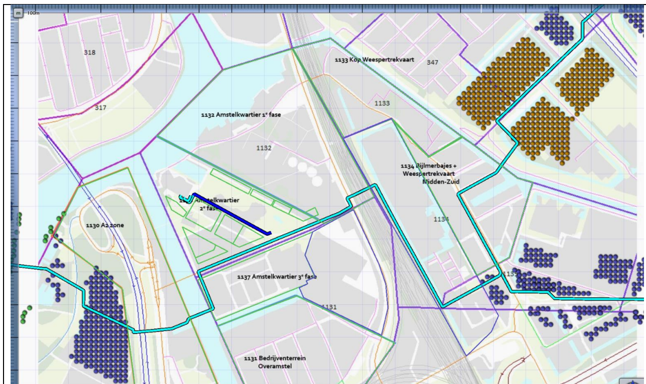
Figuur 3: ligging van de hoge druk aardgasleidingen in het plangebied.
