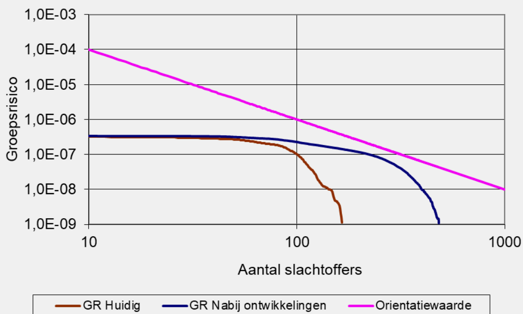
Figuur 19: Groepsrisicocurve bij het plangebied, huidige en toekomstige situatie, 4371_leiding-W-534-01-deel-1_incl, stationing 1460.
