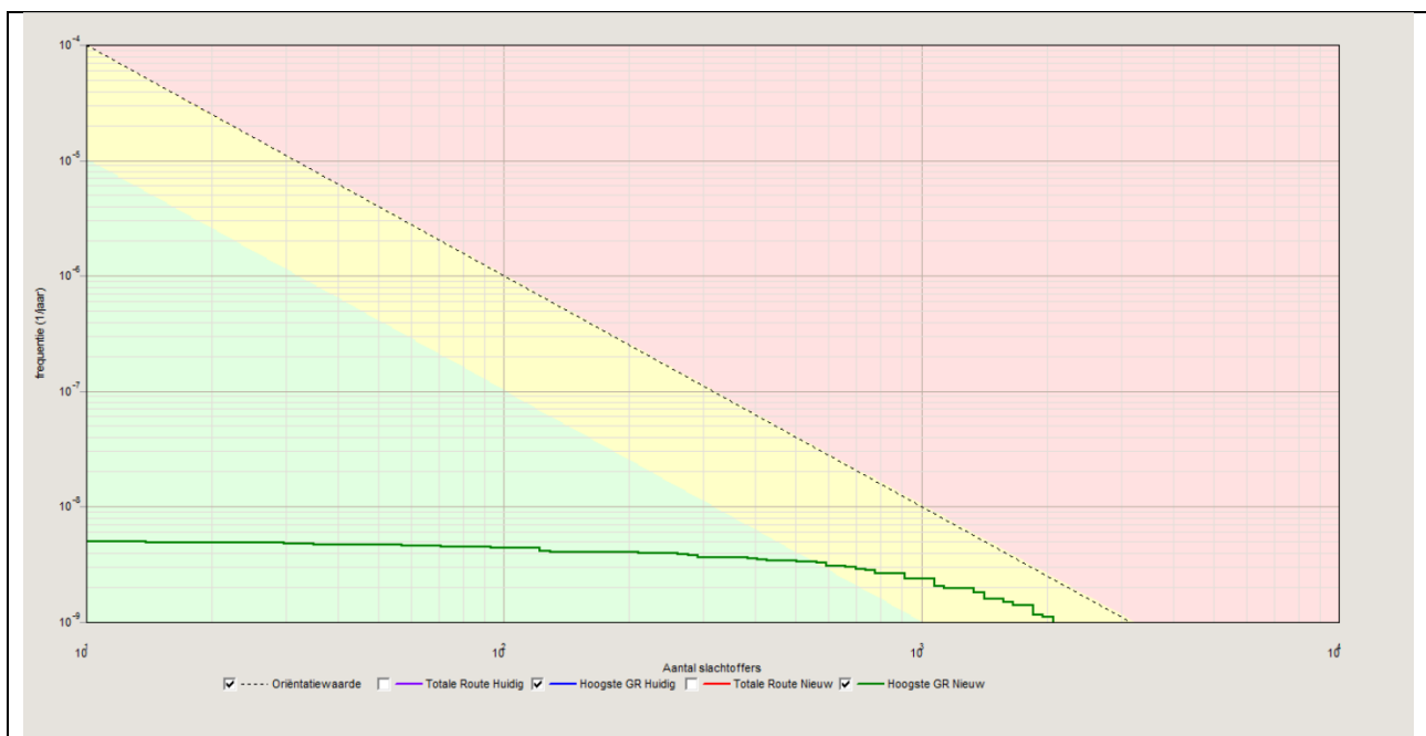
Figuur 28: Groepsrisicocurve weg, hoogste groepsrisico per kilometer, huidige en nieuwe situatie.
