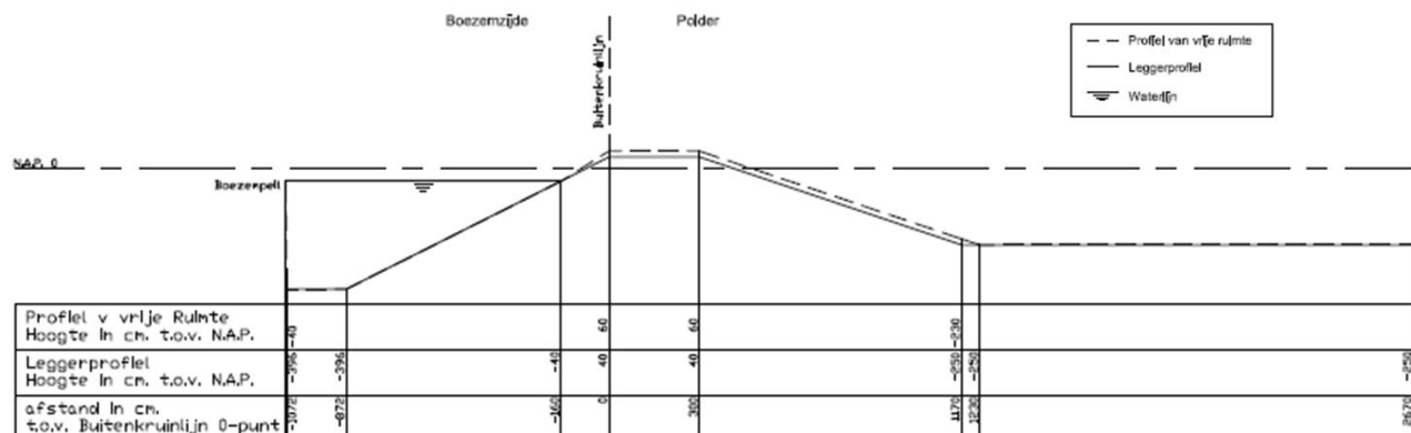
Figuur 4-3: Leggerprofiel van de waterkering
