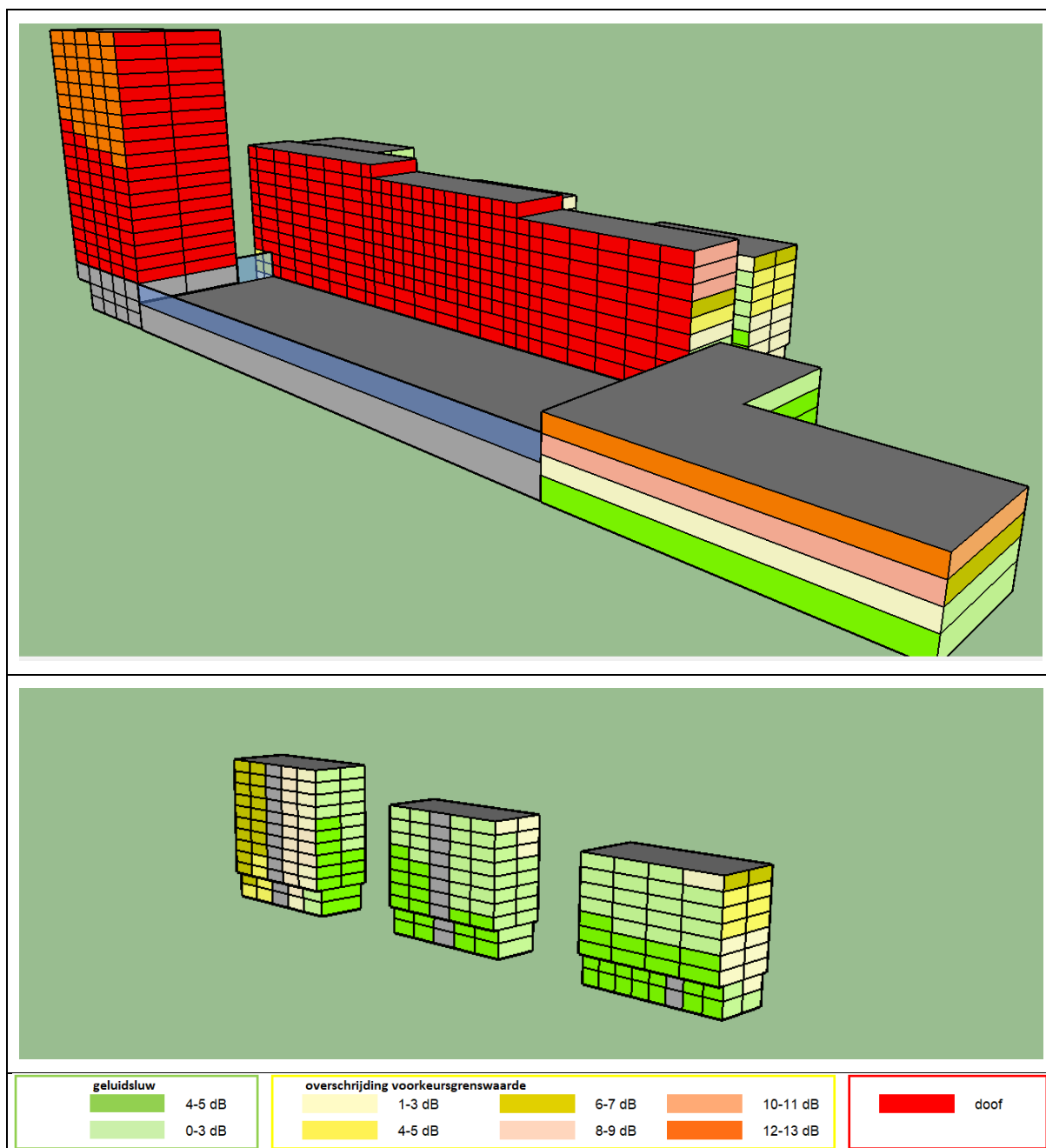
Figuur 6.1: Overzicht dove gevels, gevels met maatgevende overschrijding voorkeursgrenswaarde en geluidsluwe gevels
