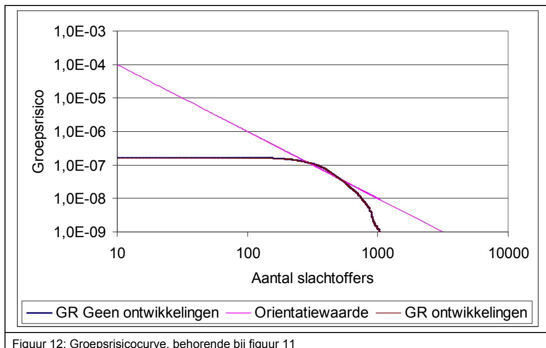
Figuur 12: Groepsrisicocurve, behorende bij figuur 11
