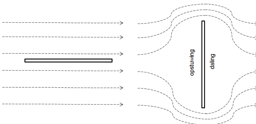
Figuur 2: Bovenaanzicht barrière; De oriëntatie van de barrière ten opzichte van de grondwaterstromingsrichting bepaalt de hinder, en daarmee de opstuwing, van het grondwater.
