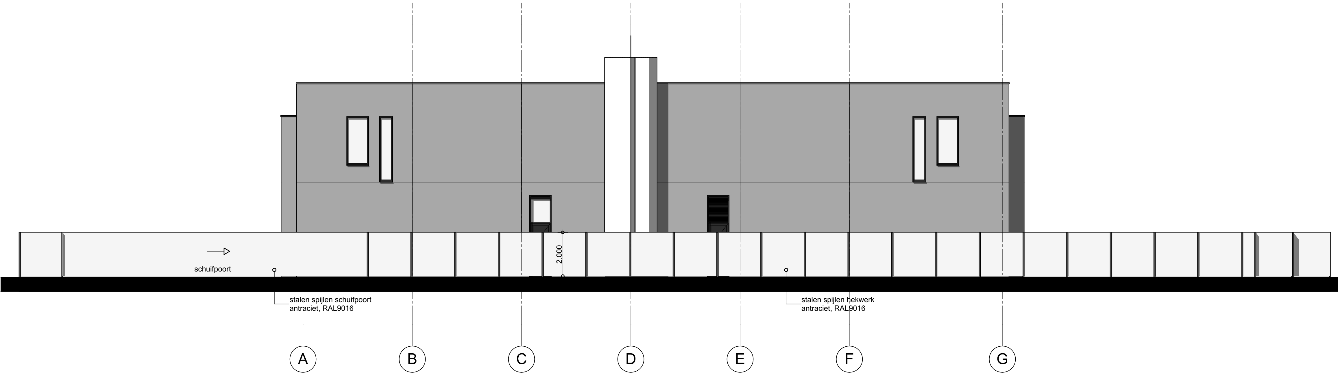
Linkergevel hekwerk
