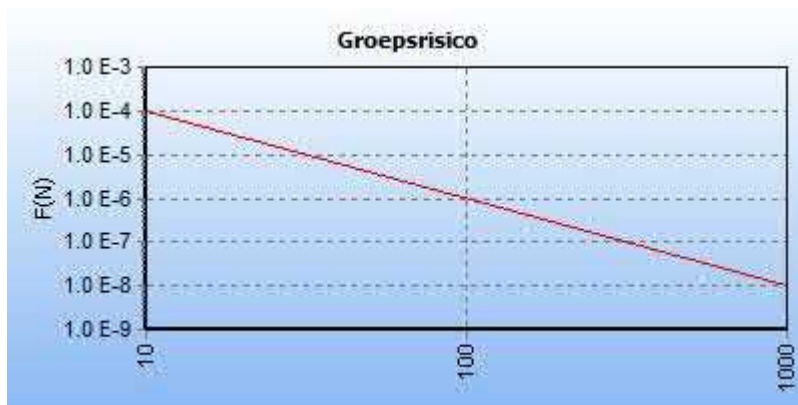
5.8 Figuur 5.8 FN curve voor 5864_leiding-W-540-03-deel-1_incl verl van N.V. Nederlandse Gasunie voor de kilometer tussen stationing 1670.00 en stationing 2360.00
