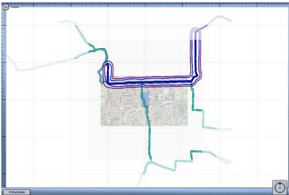
3.3 Figuur 3.3 Plaatsgebonden risico voor 5937_leiding-W-534-01-deel-1 van N.V. Nederlandse Gasunie
