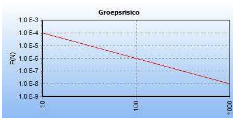
5.5 Figuur 5.5 FN curve voor 5937_leiding-W-540-03-deel-1_excl verl van N.V. Nederlandse Gasunie voor de kilometer tussen stationing 1430.00 en stationing 1930.00
