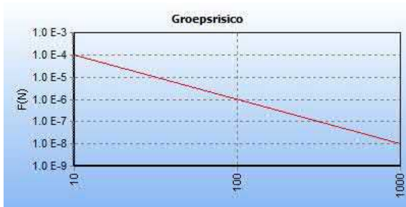
5.6 Figuur 5.6 FN curve voor 5944_leiding-W-540-03-deel-1_incl verl van N.V. Nederlandse Gasunie voor de kilometer tussen stationing 0.00 en stationing 1000.00
