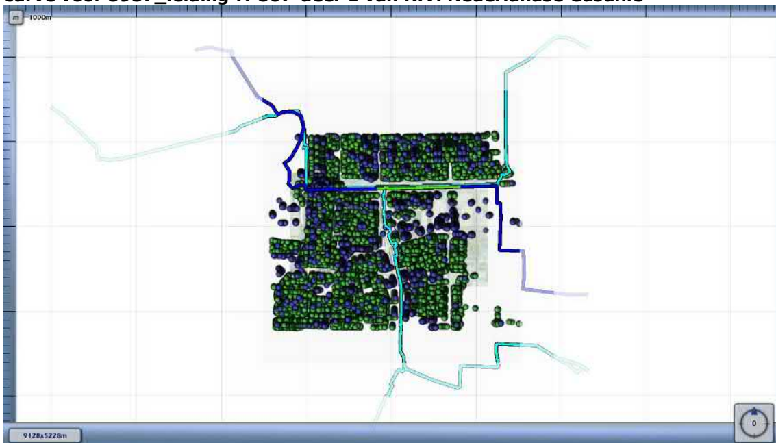
Figuur 4.2 Kilometer leiding behorende bij de maximale overschrijding van de FN-curve voor 5937_leiding-A-807-deel-1 van N.V. Nederlandse Gasunie
