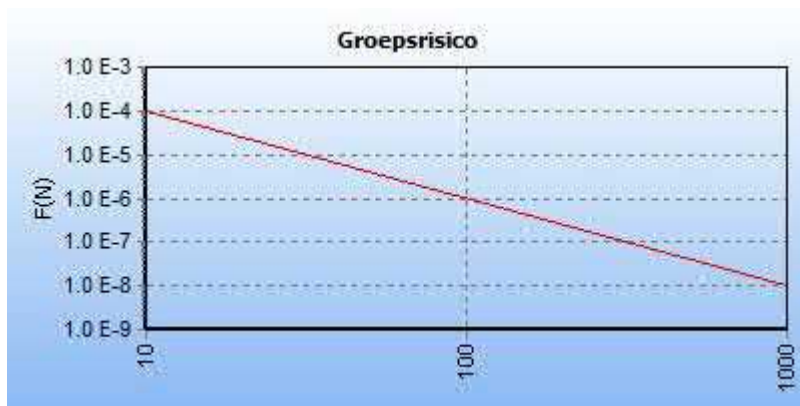
5.4 Figuur 5.4 FN curve voor 5855_leiding-W-534-01-deel-3 van N.V. Nederlandse Gasunie voor de kilometer tussen stationing 0.00 en stationing 0.00
