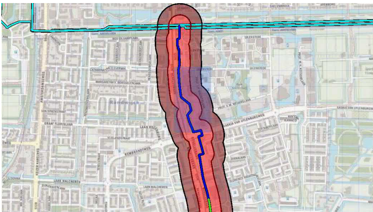
Figuur 8 - Invloedsgebied leiding W-540-01
