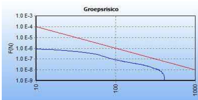
5.4 Figuur 5.4 FN curve voor 5937_leiding-W-540-01-deel-1 van N.V. Nederlandse Gasunie voor de kilometer tussen stationing 1900.00 en stationing 2900.00
