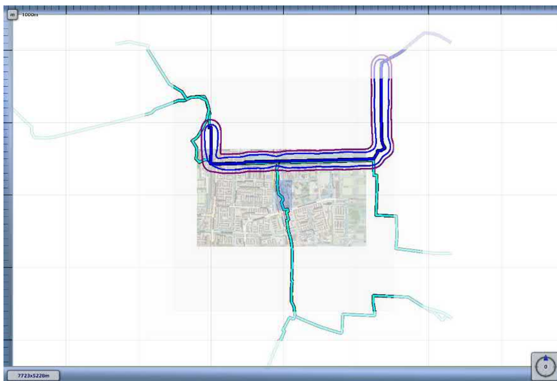
Figuur 4 - Plaatsgebonden risicocontouren leiding W-534-01
