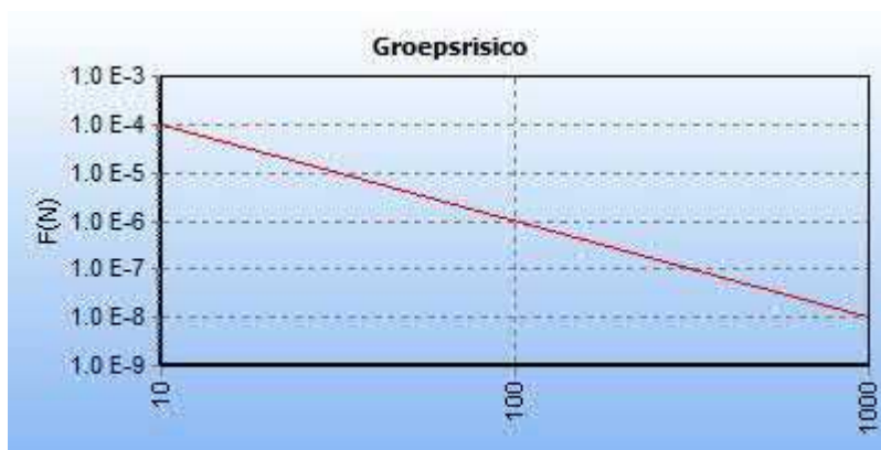
5.8 Figuur 5.8 FN curve voor 5864_leiding-W-540-03-deel-1_incl verl van N.V. Nederlandse Gasunie voor de kilometer tussen stationing 1670.00 en stationing 2360.00
