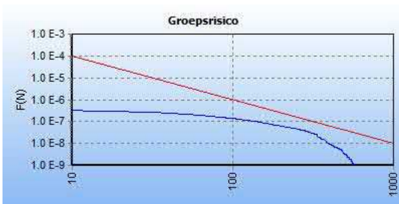
5.2 Figuur 5.2 FN curve voor 5855_leiding-W-534-01-deel-1 van N.V. Nederlandse Gasunie voor de kilometer tussen stationing 22210.00 en stationing 23210.00
