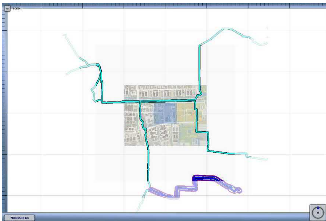
3.7 Figuur 3.7 Plaatsgebonden risico voor 5855_leiding-W-540-03-deel-1_excl verl van N.V. Nederlandse Gasunie
