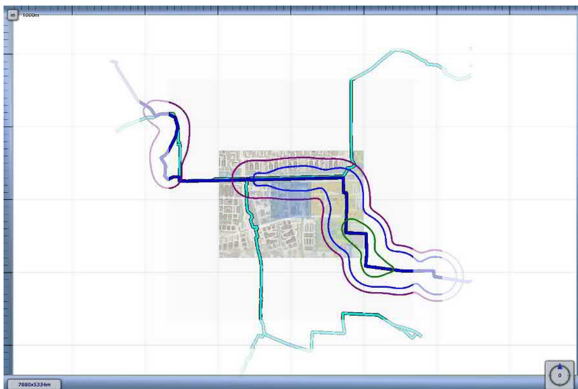
3.1 Figuur 3.1 Plaatsgebonden risico voor 5855_leiding-A-807-deel-1 van N.V. Nederlandse Gasunie
