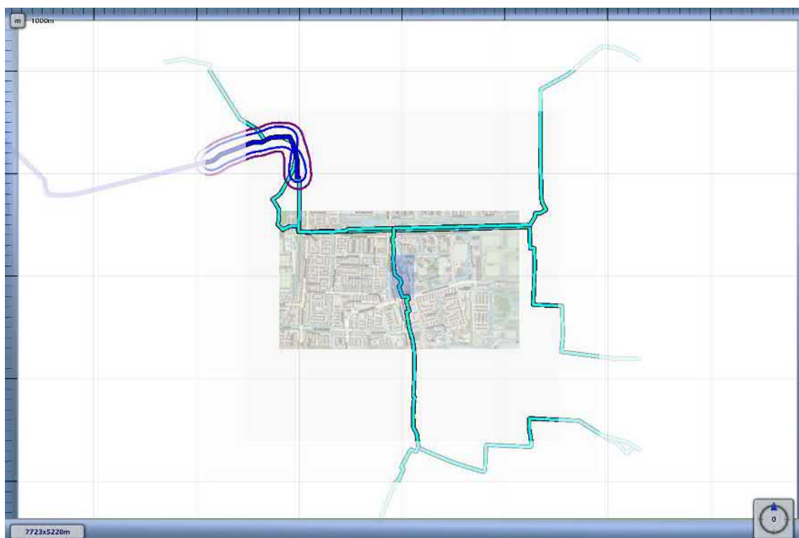
3.1 Figuur 3.1 Plaatsgebonden risico voor 5918_leiding-W-534-01-deel-3_6_2_7bis van N.V. Nederlandse Gasunie
