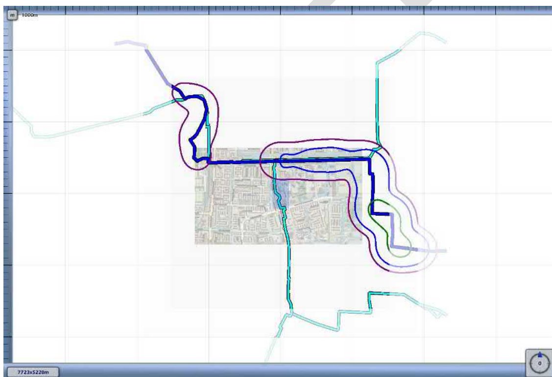
Figuur 3 - Plaatsgebonden risicocontouren leiding A-807
