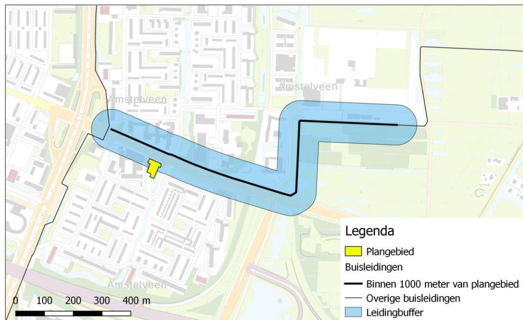
Figuur 2. Aardgasleiding W540-03 en invloedsgebied
