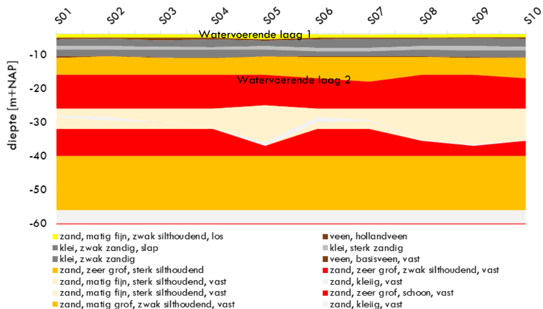
figuur 2 – schematisering bodem
