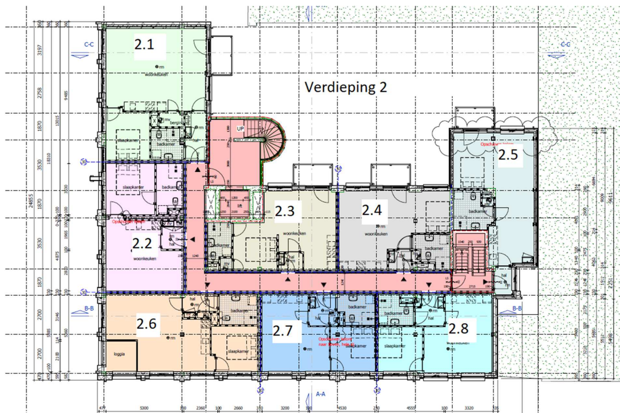
Figuur 2: Plattegrond verdieping 2
