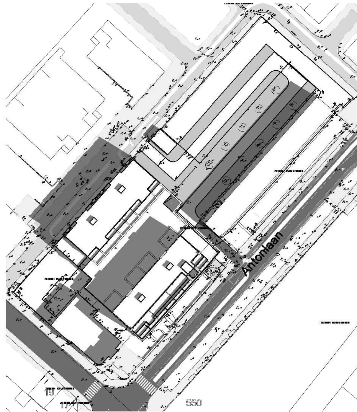
2 | bezonning 21-09 12.00h 1 : 1000
