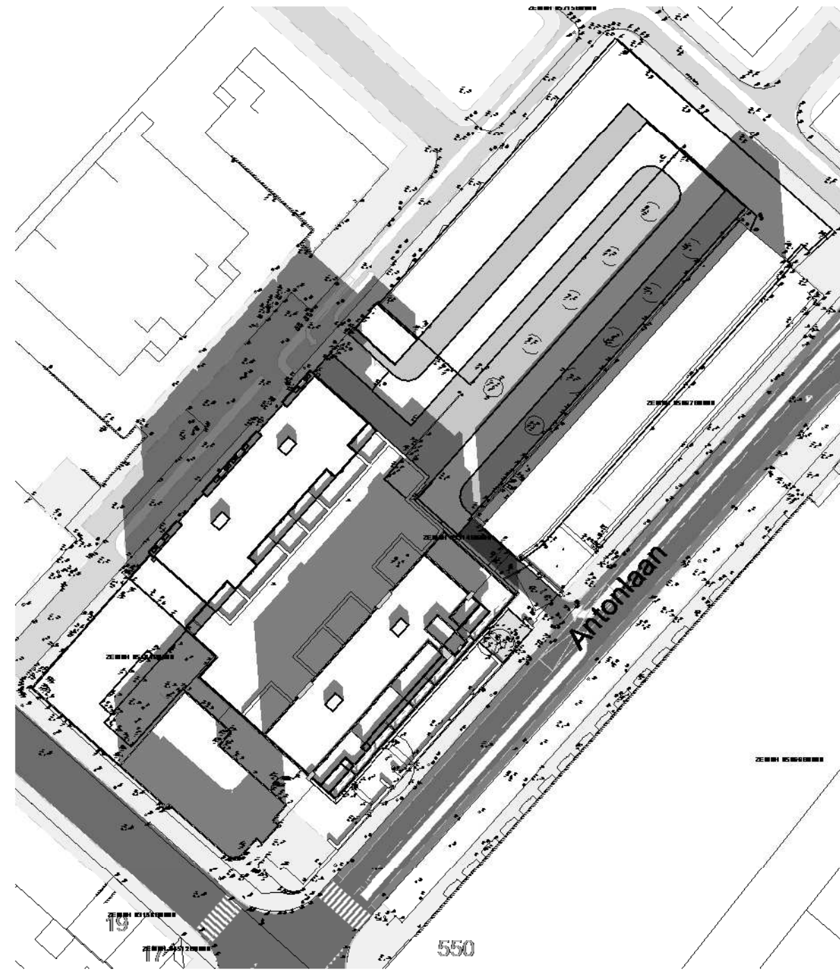
3 | bezonning 21-09 15.00h 1 : 1000
