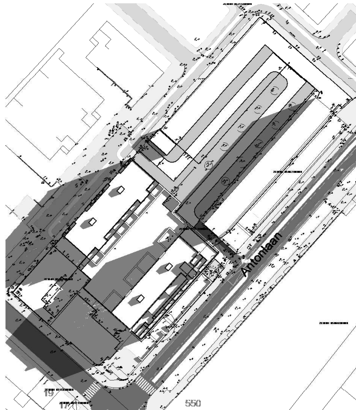
1 bezonning 21-03 9.00h 1 : 1000
