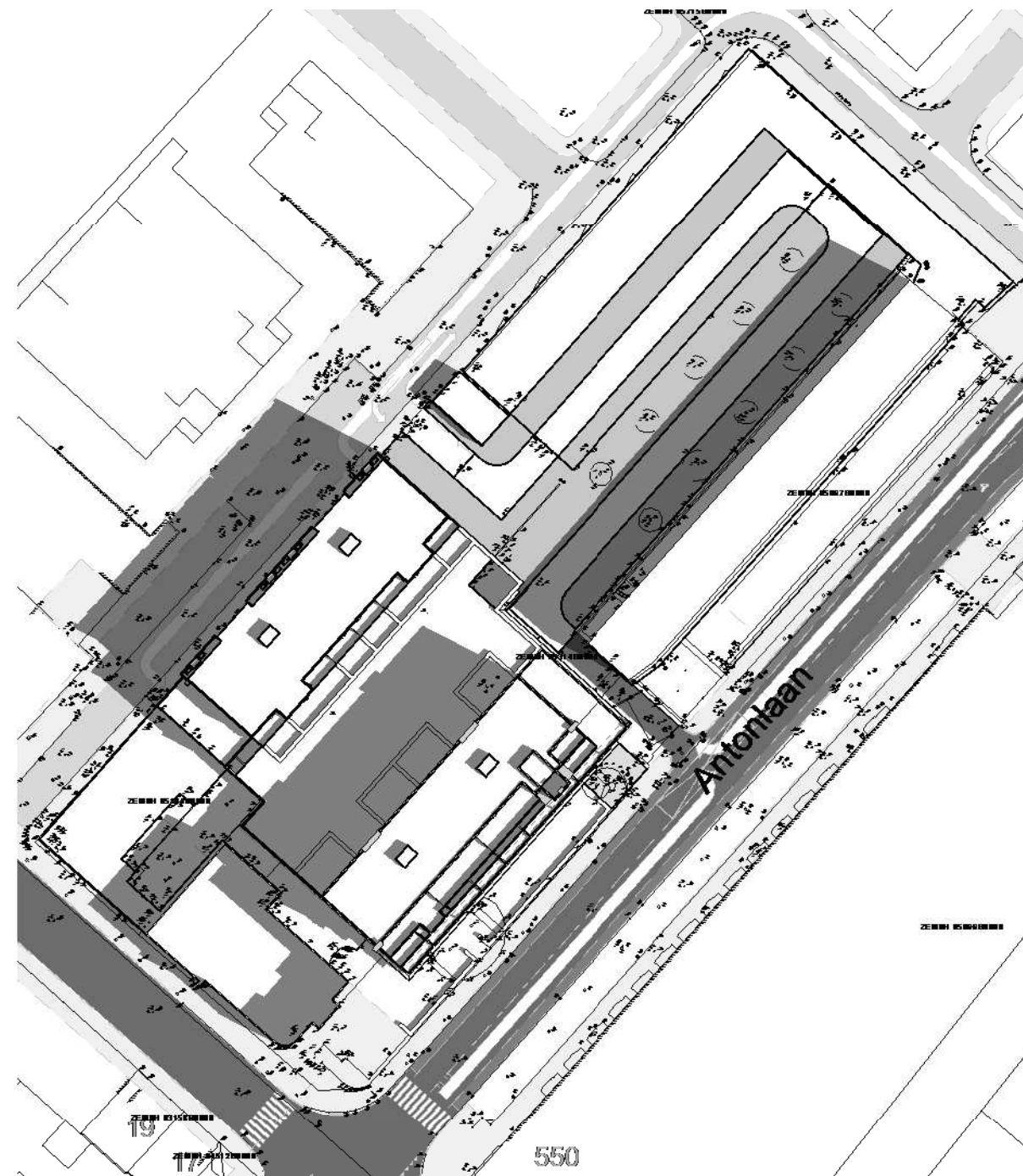
2 bezonning 21-03 12.00h 1 : 1000
