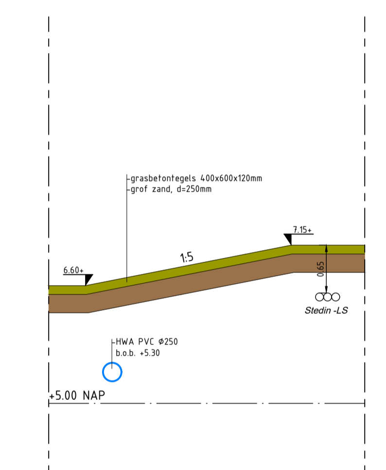
Doorsnede F-F Schaal 1:50
