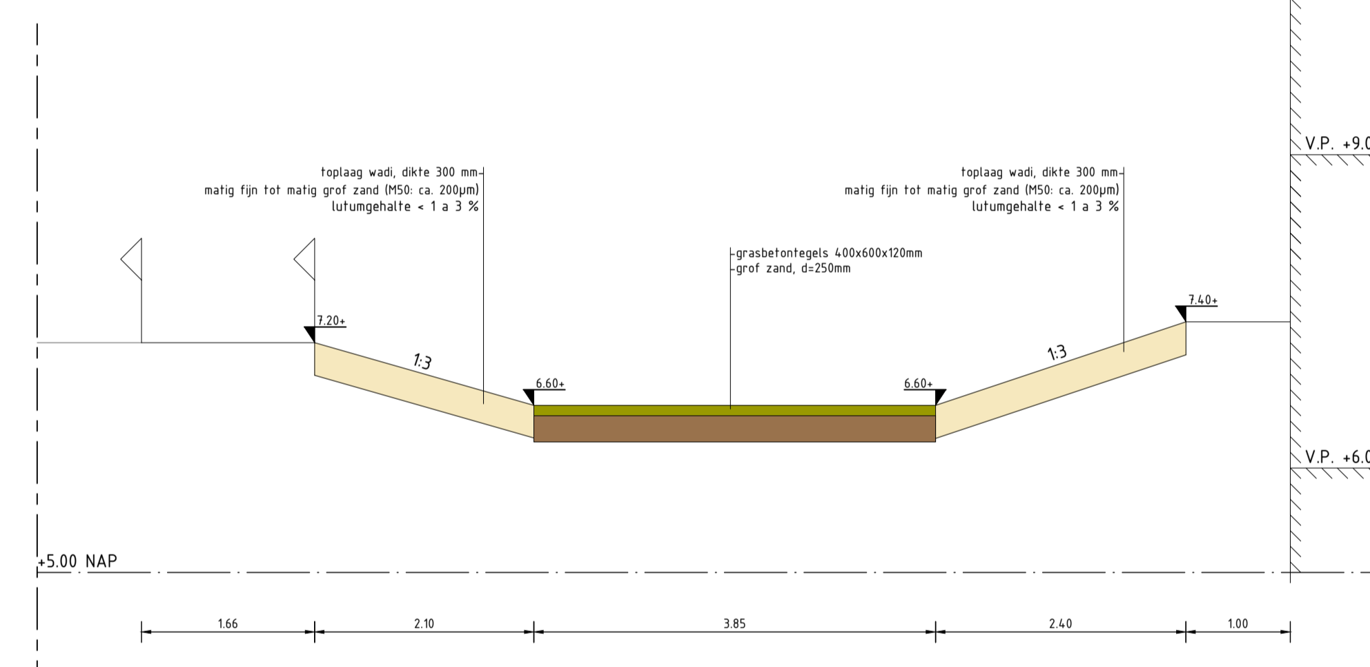
Doorsnede E-E Schaal 1:50
