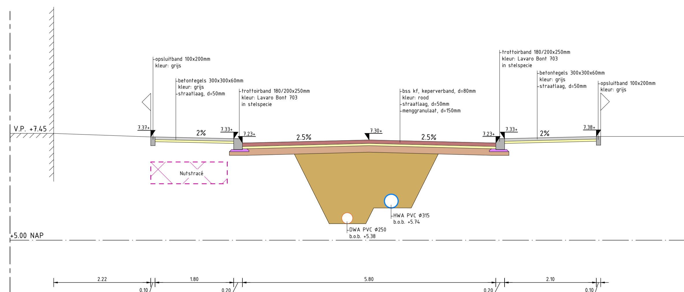
Doorsnede C-C Schaal 1:50
