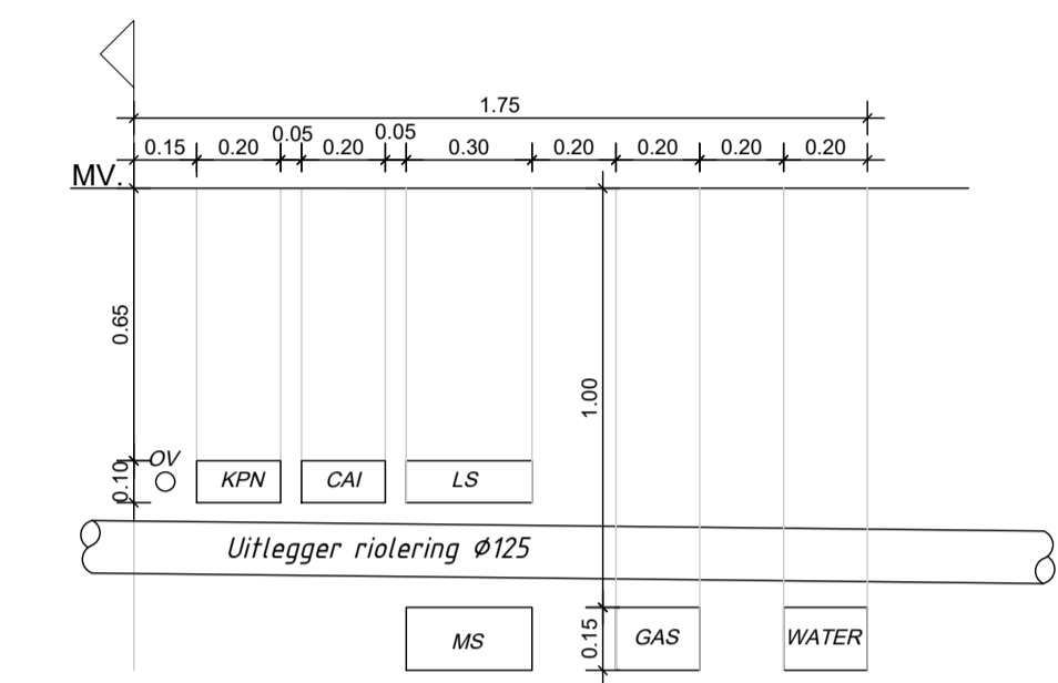
Principeprofiel nuts 1.75m Schaal 1:20
