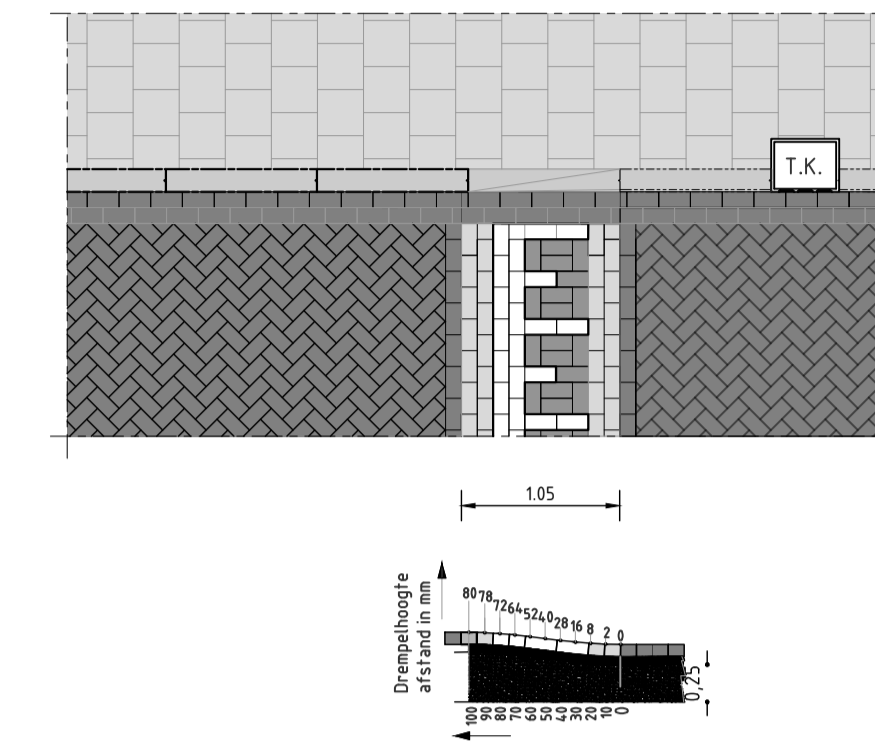
Detail plateau Schaal 1:50
