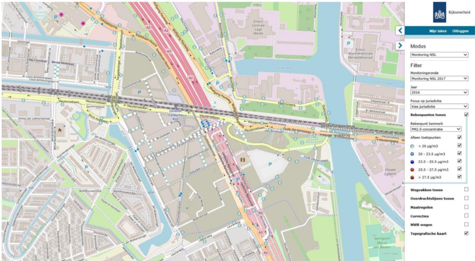
Afbeelding 3: Concentraties uit NSL-Monitoringstool voor PM2,5 voor het jaar 2016
