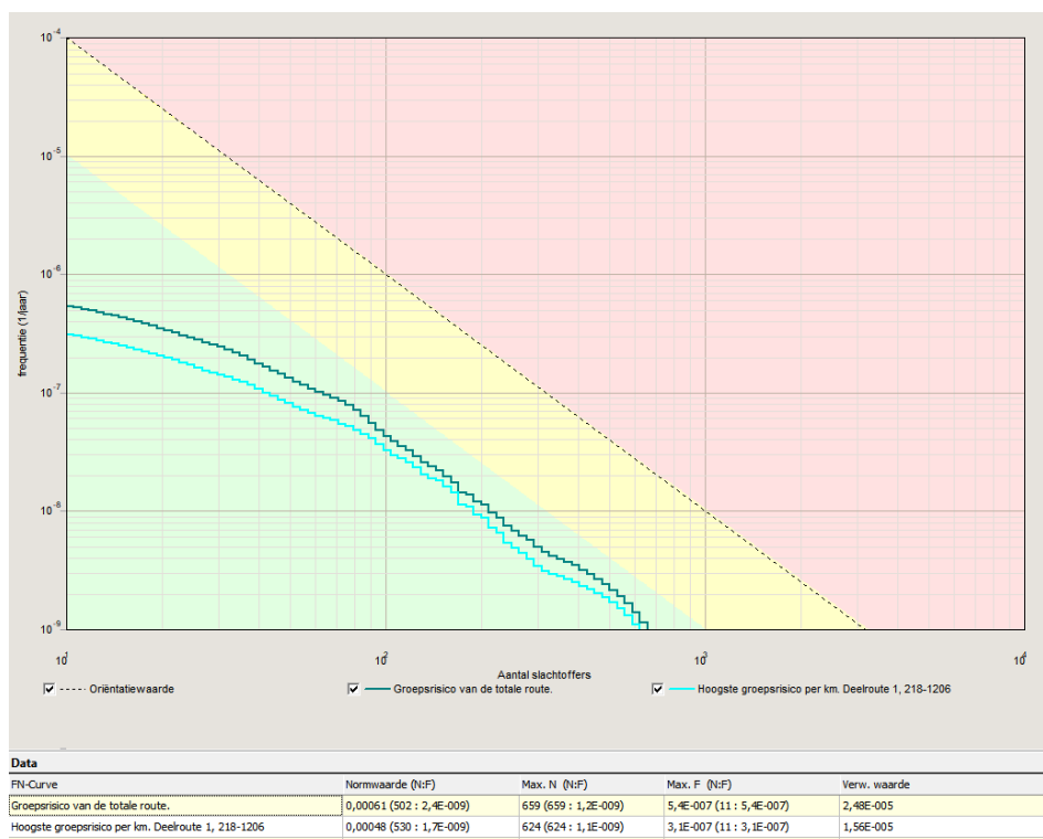
Afbeelding 4 fN-curve berekend groepsrisico, toekomstige situatie
