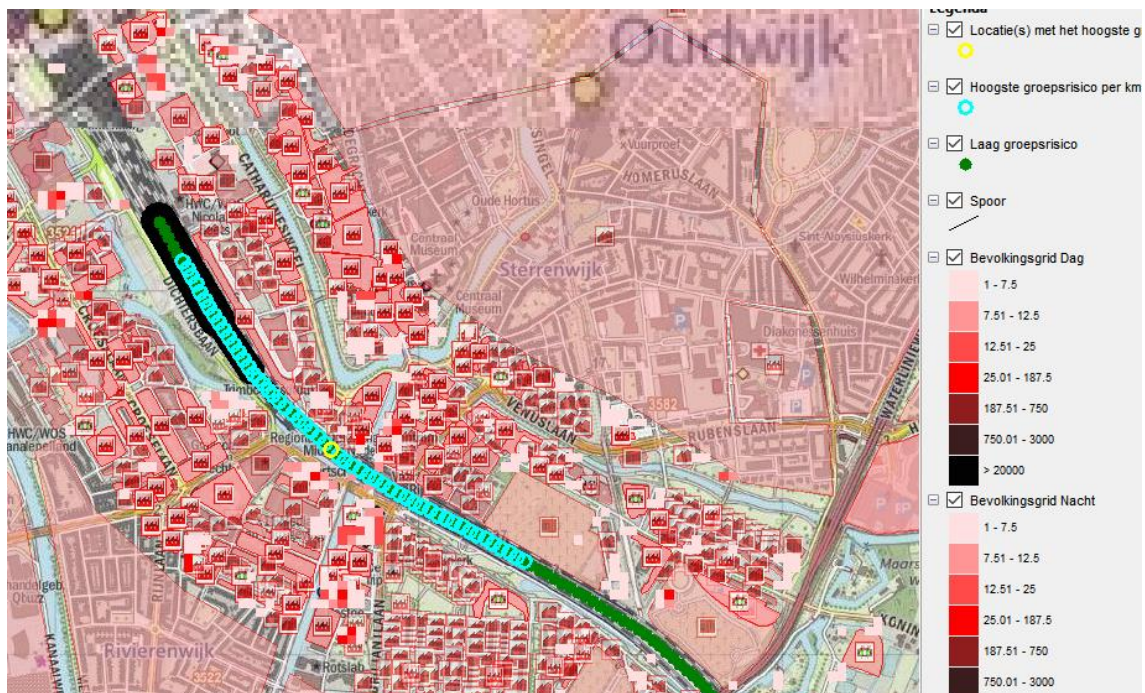
Afbeelding 3 Locatie met hoogste GR spoor - huidige situatie
