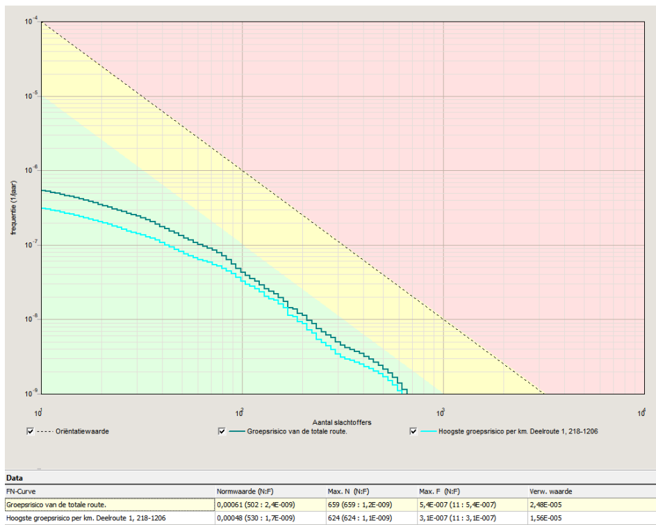
Afbeelding 2 fN-curve berekend groepsrisico - huidige situatie
