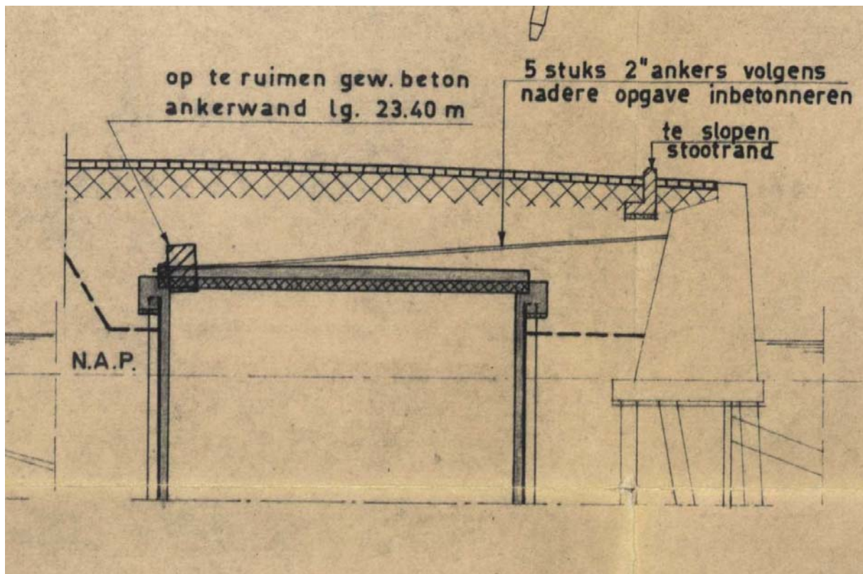
Afbeelding 8 Doorsnede F-F
