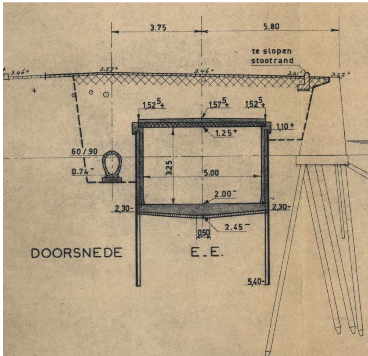
Afbeelding 7 Doorsnede E-E
