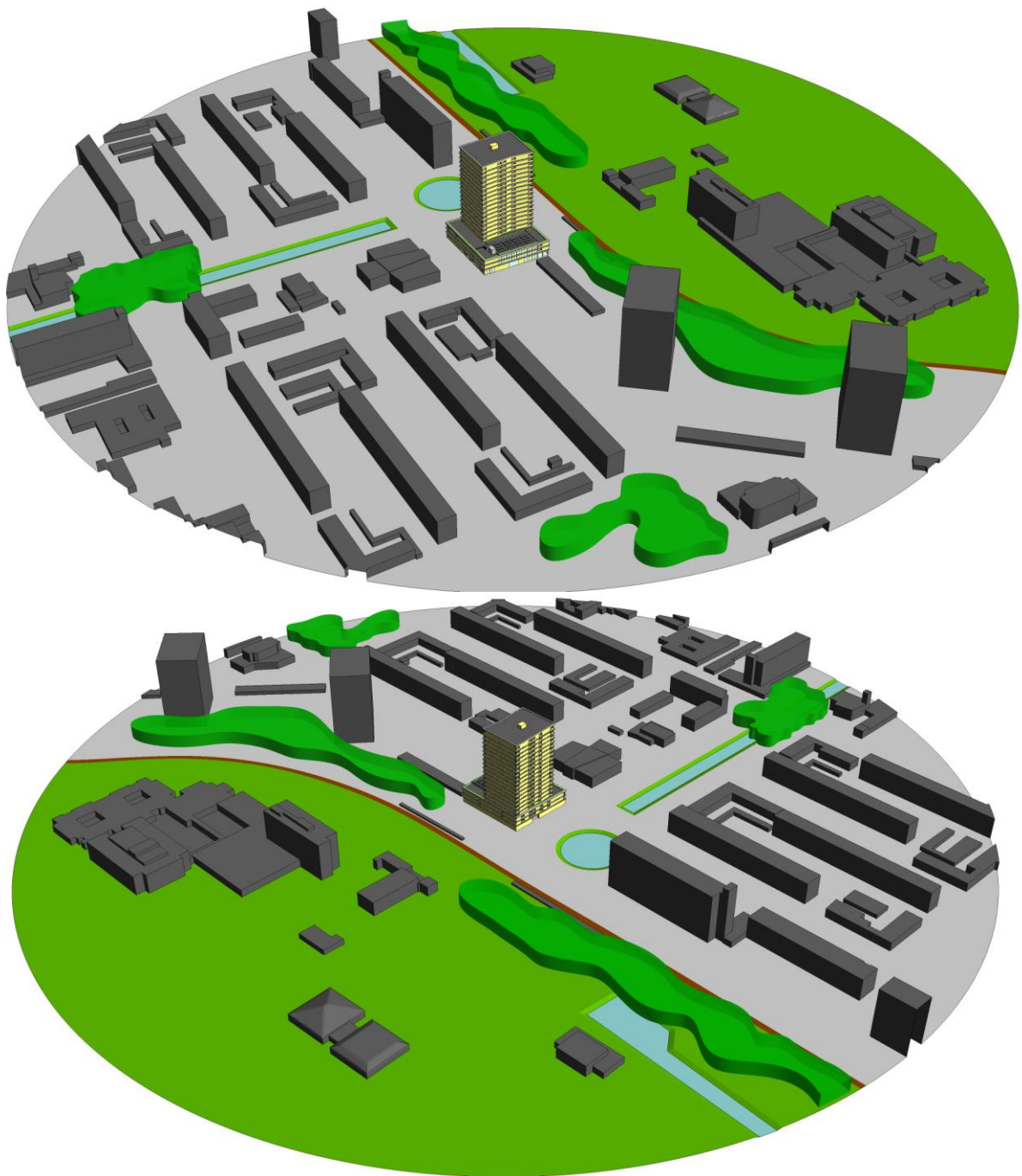
Figuur 2: Overzicht van het 3D CFD model met omliggende bebouwing.
