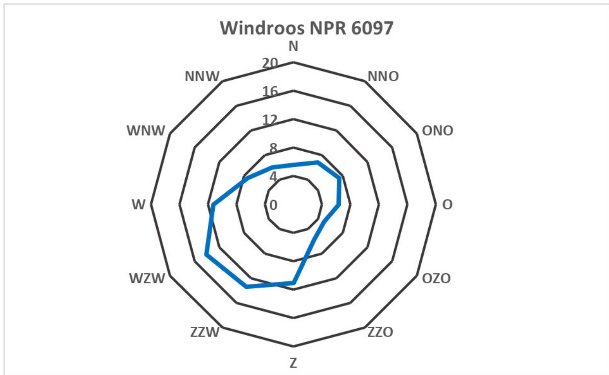
Figuur 3: Windroos Beneluxlaan Utrecht, volgens NPR 6097.
