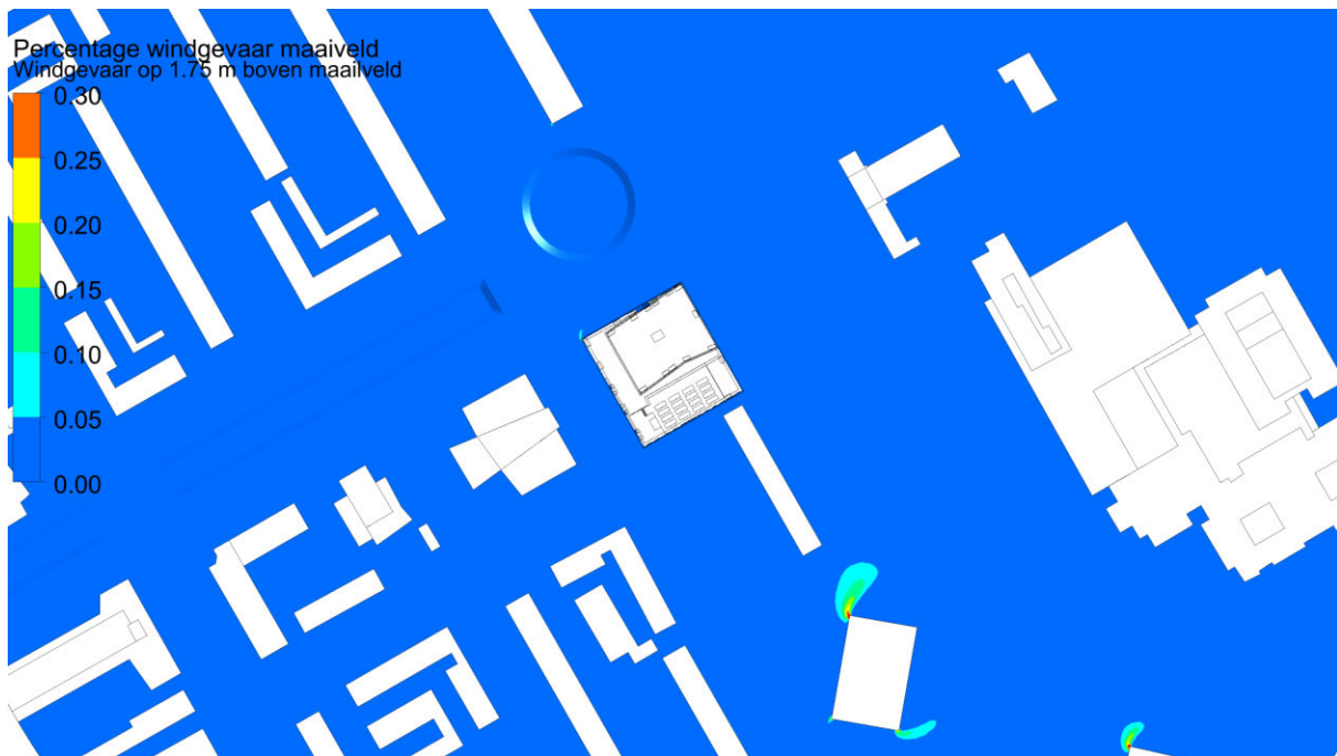
Figuur 9: Percentage windgevaar per jaar op 1,75 m boven maaiveld.
