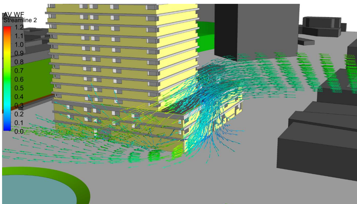
Figuur 8: Stroomlijnen van de lucht die langs de woontoren naar beneden wordt geduwd en versnelt op maaiveldniveau voor windrichting 240 (WZW).
