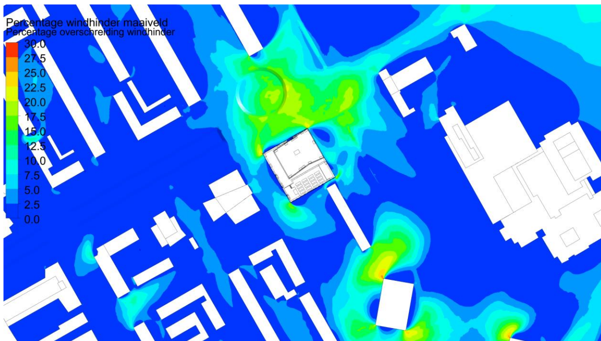
Figuur 7: Percentage windhinder op 1,75 m boven het maaiveld.
