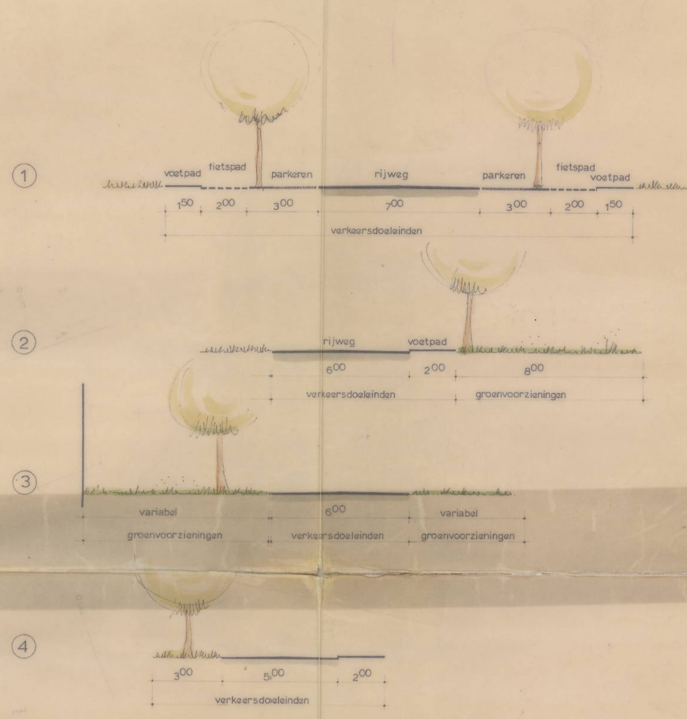
DWARSPROFIELEN 1:100
