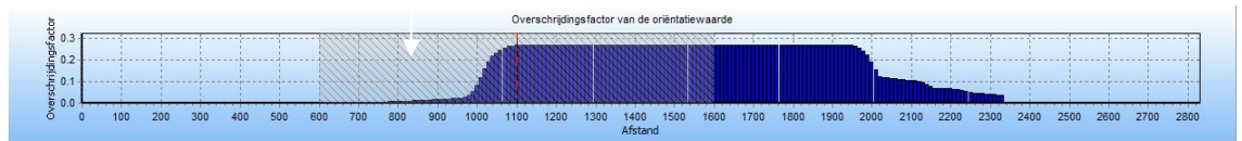
Figuur 2.3: Groepsrisico screening W-520-06-deel-1, voor planrealisatie
