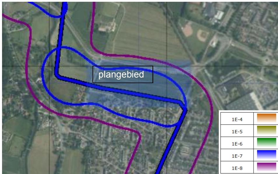
Figuur 2.2: Uitsnede CAROLA plaatsgebonden risico voor leiding W-520-06-deel-1
