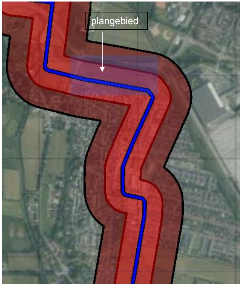
Figuur 2.1: Uitsnede CAROLA invloedsgebied buisleiding
