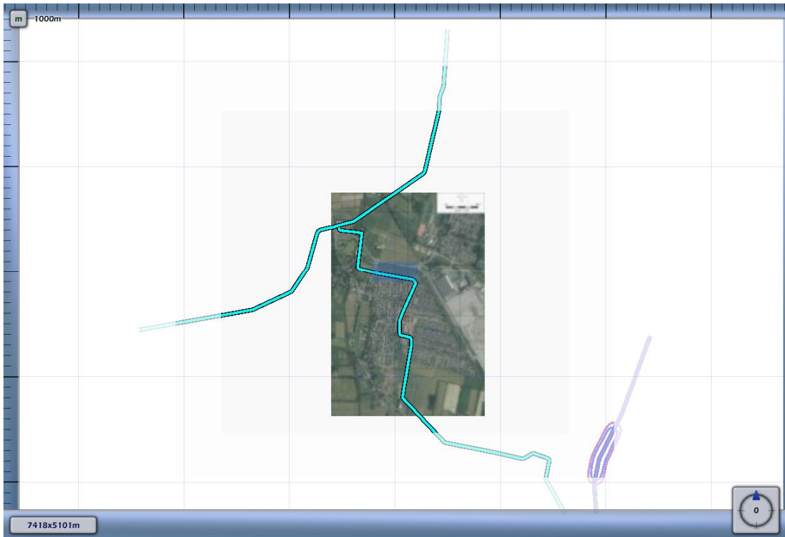
3.3 Figuur 3.3 Plaatsgebonden risico voor 5322_leiding-W-520-06-deel-1 van N.V. Nederlandse Gasunie
