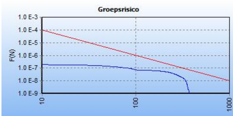
5.2 Figuur 5.2 FN curve voor 4436_leiding-W-520-01-deel-1 van N.V. Nederlandse Gasunie voor de kilometer tussen stationing 0.00 en stationing 0.00
