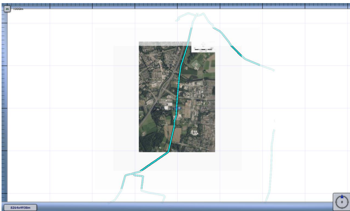
3.4 Figuur 3.4 Plaatsgebonden risico voor 4436_leiding-W-520-05-deel-1 van N.V. Nederlandse Gasunie
