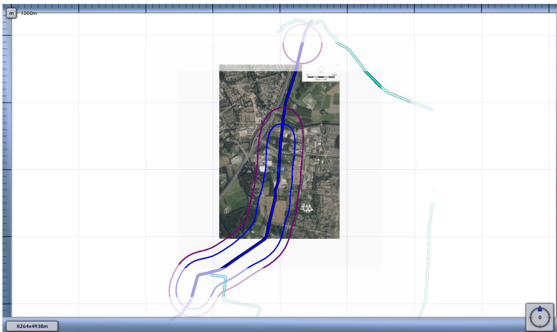
3.2 Figuur 3.2 Plaatsgebonden risico voor 4436_leiding-W-520-01-deel-1 van N.V. Nederlandse Gasunie
