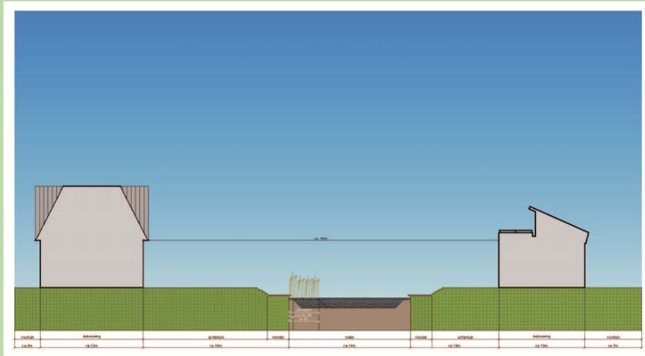
Figuur 3.2 Profiel watergang tussen bestaande woningen Zilverdijk en nieuwe woningen deelplan 1.3
