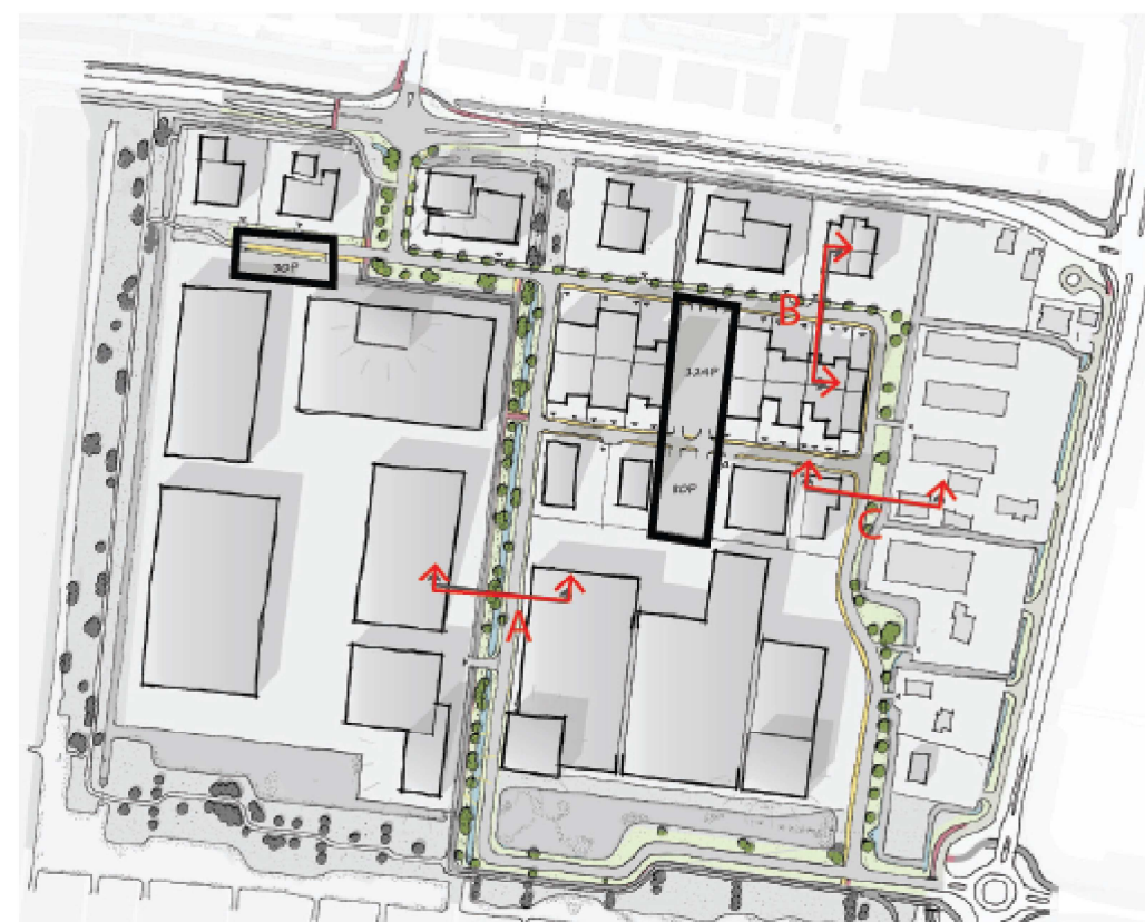
Locaties parkeren openbare ruimte en dwarsprofielen
