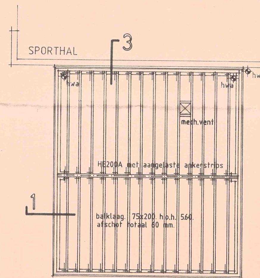
platbalklaag
