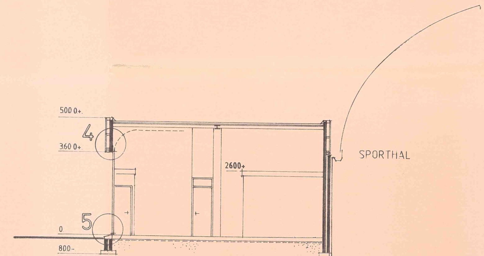
doorsnede A
