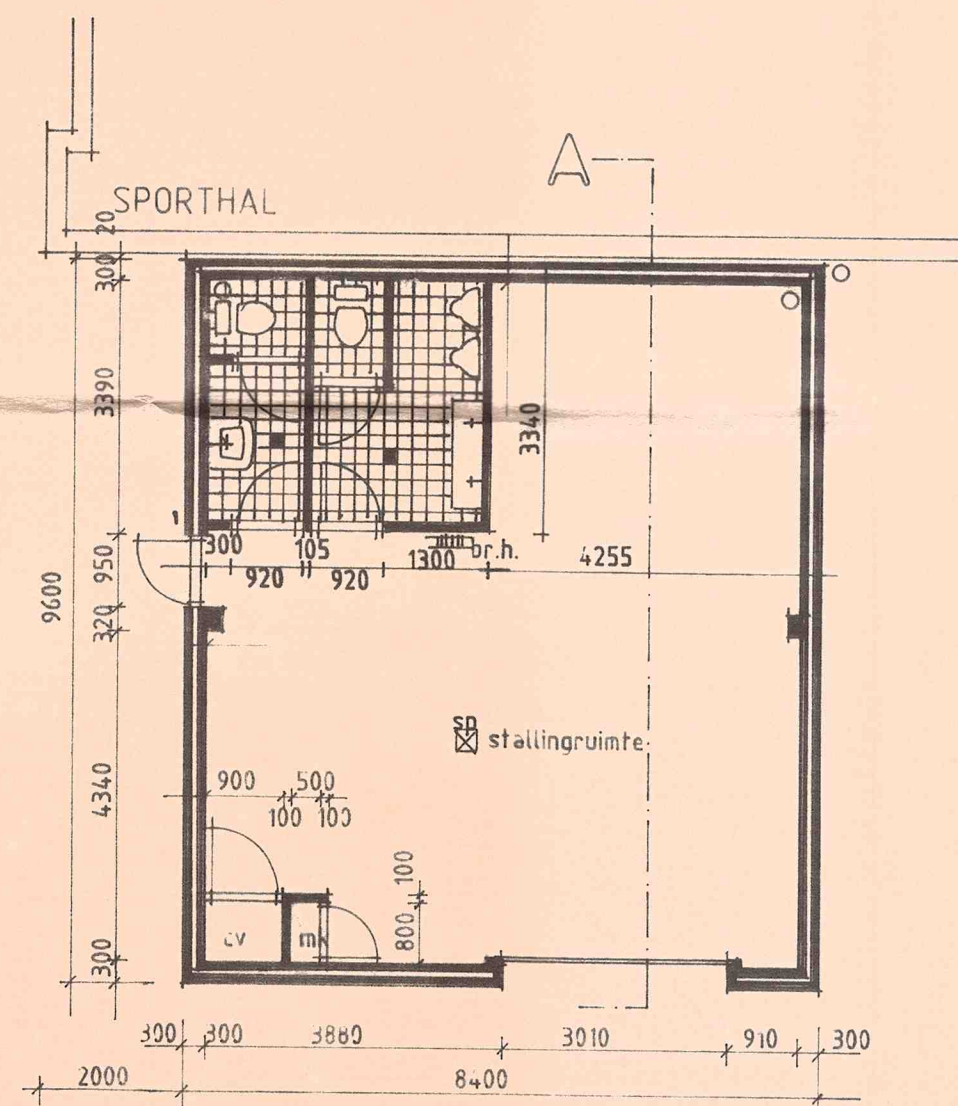
plattegrond
