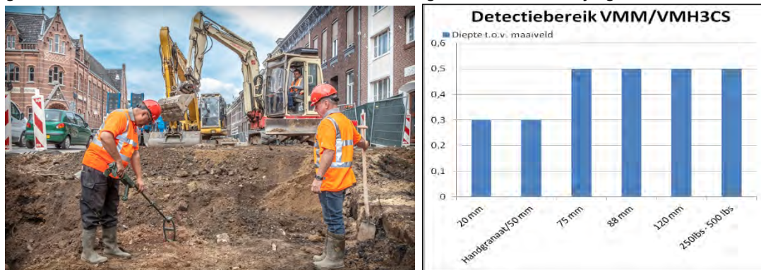
Figuur 7. Uitvoeren actieve realtime oppervlakedetectie m.b.v. Vallon VMM/ VMH3CS non Ferrous Locator en staafdiagram waarop het maximale detectiebereik (m 1 – mv) per kaliber is aangegeven.
