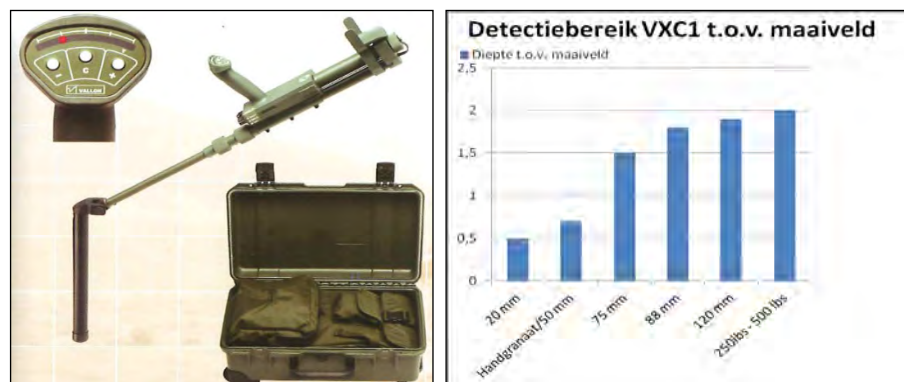
Figuur 5. Vallon VXC1 Ferrous Locator (magnetometer) welke geschikt is voor passieve realtime oppervlakedetectie en staafdiagram waarop het maximale detectiebereik ( m^2 - mv ) per kaliber is aangegeven.
