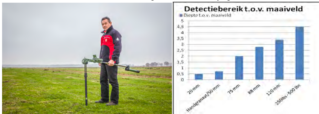
Figuur 4. Passieve realtime oppervlakedetectie met VX1 Ferrous Locator (magnetometer) en staafdiagram waarop het maximale detectiebereik ( m^2 - mv ) per kaliber is aangegeven.
