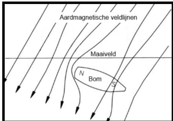
Figuur 3. Principe weergave werking passieve realtime oppervlakedetectie/ magnetometrie.
