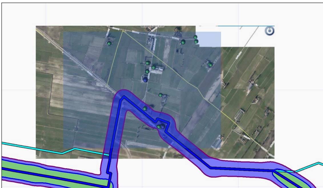
3.2 Figuur 3.2 Plaatsgebonden risico voor 3493_leiding-W-500-01-deel-1 van N.V. Nederlandse Gasunie
