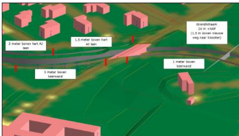
Figuur 43 Maatregel: afscherming
