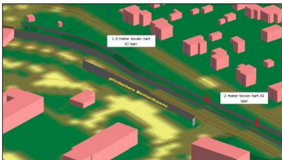
Figuur 41 Maatregel: afscherming
