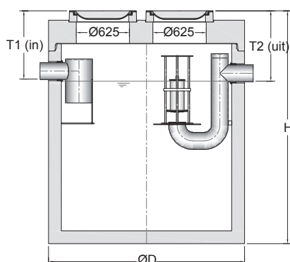
Dwarsdoorsnede
