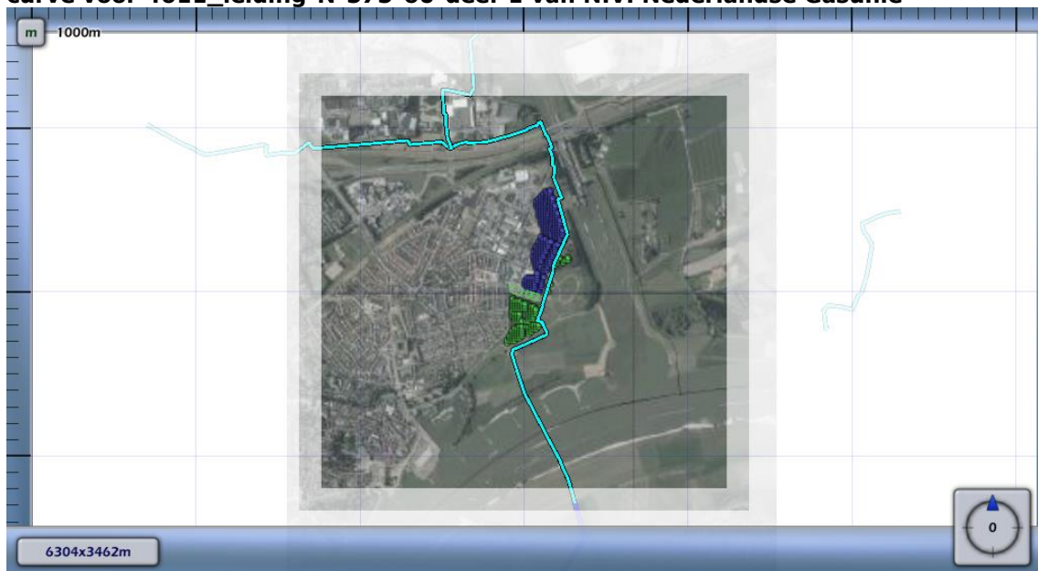
Figuur 4.4 Kilometer leiding behorende bij de maximale overschrijding van de FN-curve voor 4611_leiding-N-575-60-deel-1 van N.V. Nederlandse Gasunie
