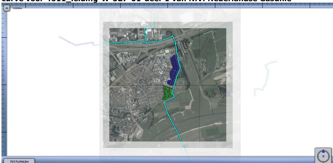
Figuur 4.7 Kilometer leiding behorende bij de maximale overschrijding van de FN-curve voor 4611_leiding-W-527-01-deel-1 van N.V. Nederlandse Gasunie
