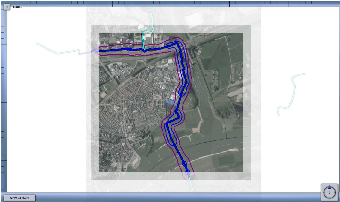
3.6 Figuur 3.6 Plaatsgebonden risico voor 4611_leiding-W-525-05-deel-1 van N.V. Nederlandse Gasunie
