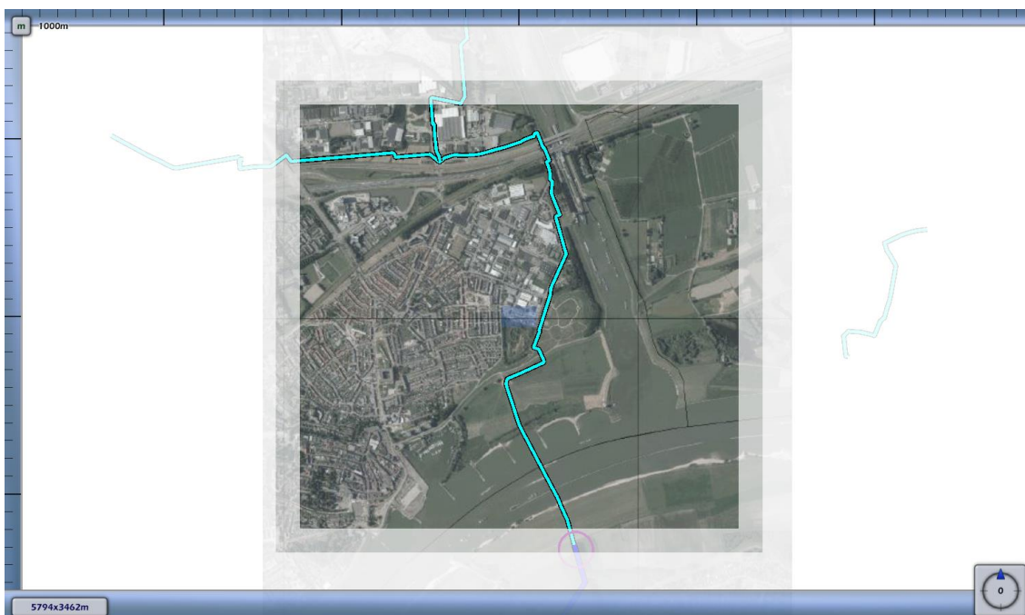
3.4 Figuur 3.4 Plaatsgebonden risico voor 4611_leiding-N-575-60-deel-1 van N.V. Nederlandse Gasunie
