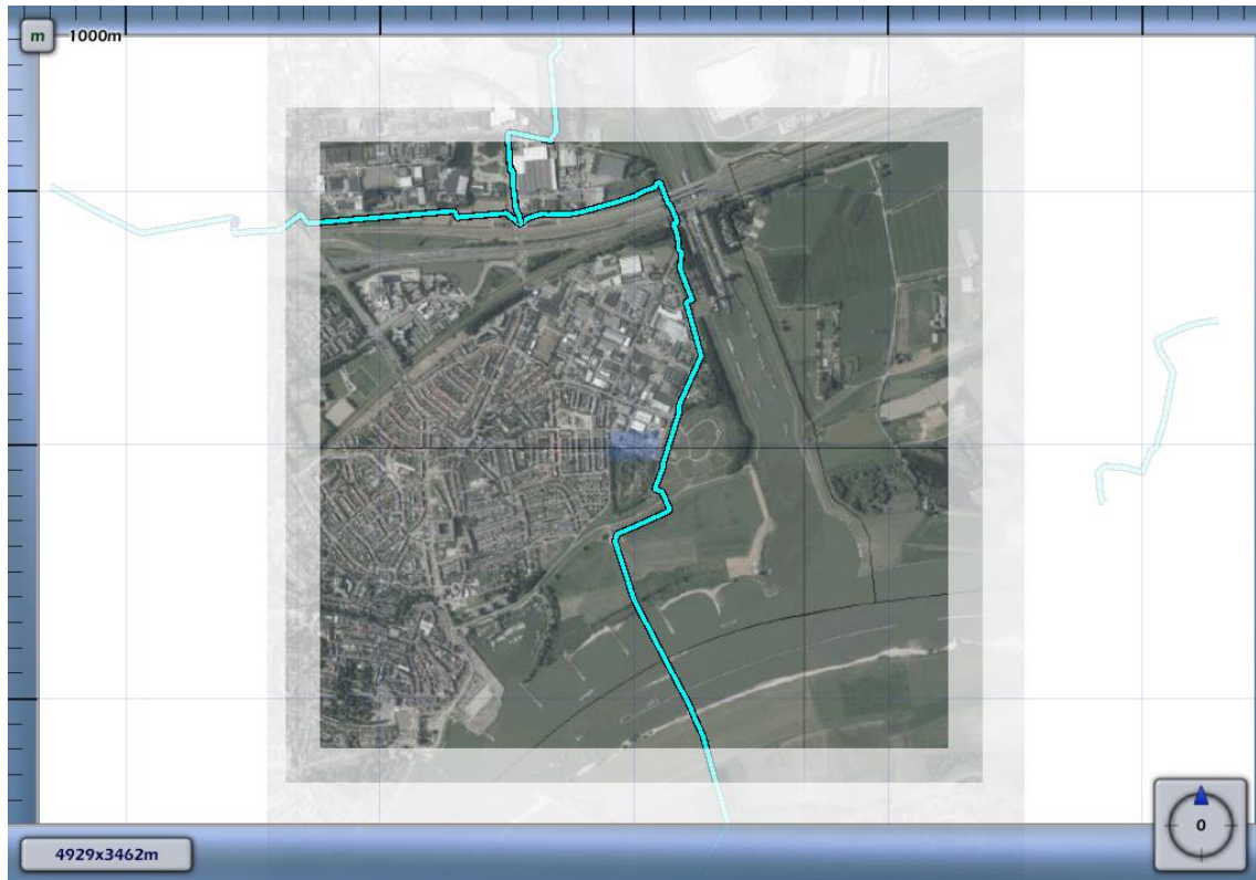
3.8 Figuur 3.8 Plaatsgebonden risico voor 4611_leiding-W-527-22-deel-1 van N.V. Nederlandse Gasunie
