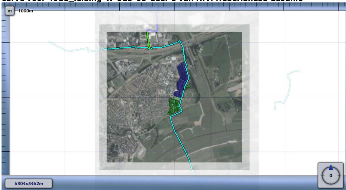
Figuur 4.6 Kilometer leiding behorende bij de maximale overschrijding van de FN-curve voor 4611_leiding-W-525-05-deel-1 van N.V. Nederlandse Gasunie
