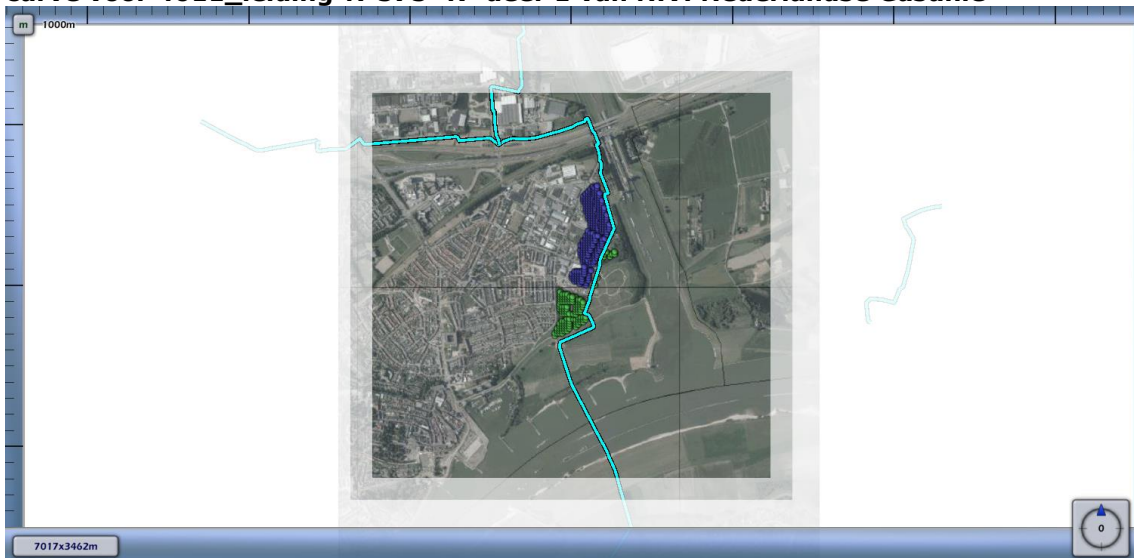
Figuur 4.3 Kilometer leiding behorende bij de maximale overschrijding van de FN-curve voor 4611_leiding-N-575-47-deel-1 van N.V. Nederlandse Gasunie
