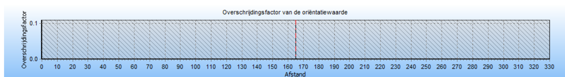
4.6 Figuur 4.6 Groepsrisico screening voor 4611_leiding-W-525-05-deel-1 van N.V. Nederlandse Gasunie
