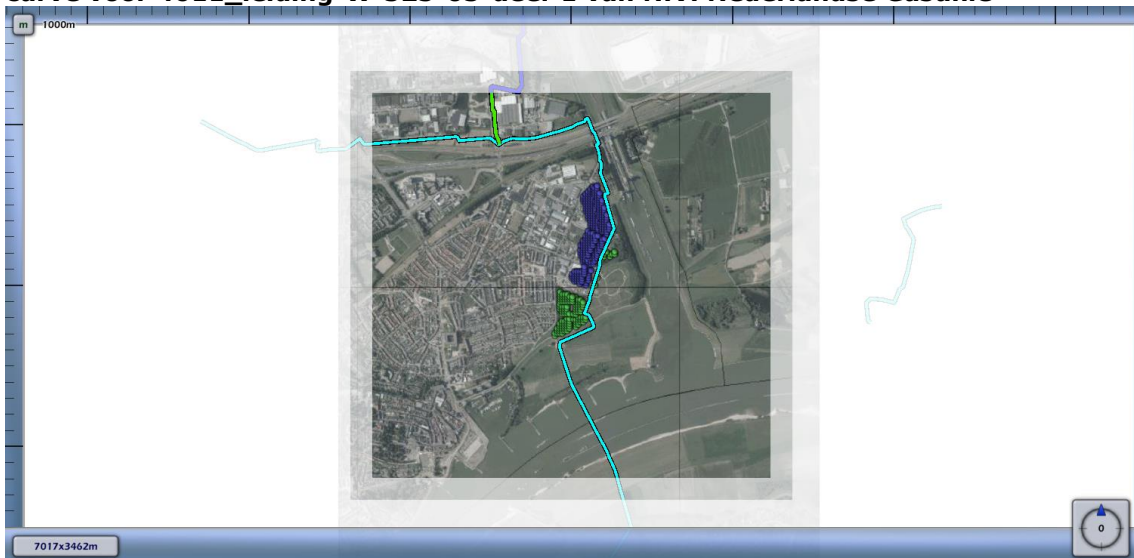
Figuur 4.6 Kilometer leiding behorende bij de maximale overschrijding van de FN-curve voor 4611_leiding-W-525-05-deel-1 van N.V. Nederlandse Gasunie
