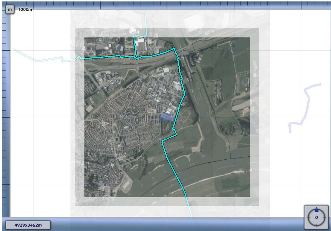
3.3 Figuur 3.3 Plaatsgebonden risico voor 4611_leiding-N-575-47-deel-1 van N.V. Nederlandse Gasunie
