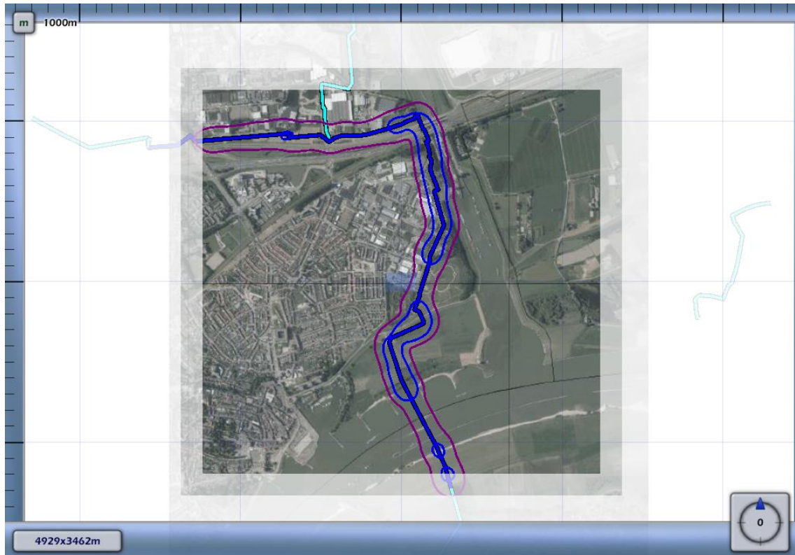
3.6 Figuur 3.6 Plaatsgebonden risico voor 4611_leiding-W-525-05-deel-1 van N.V. Nederlandse Gasunie
