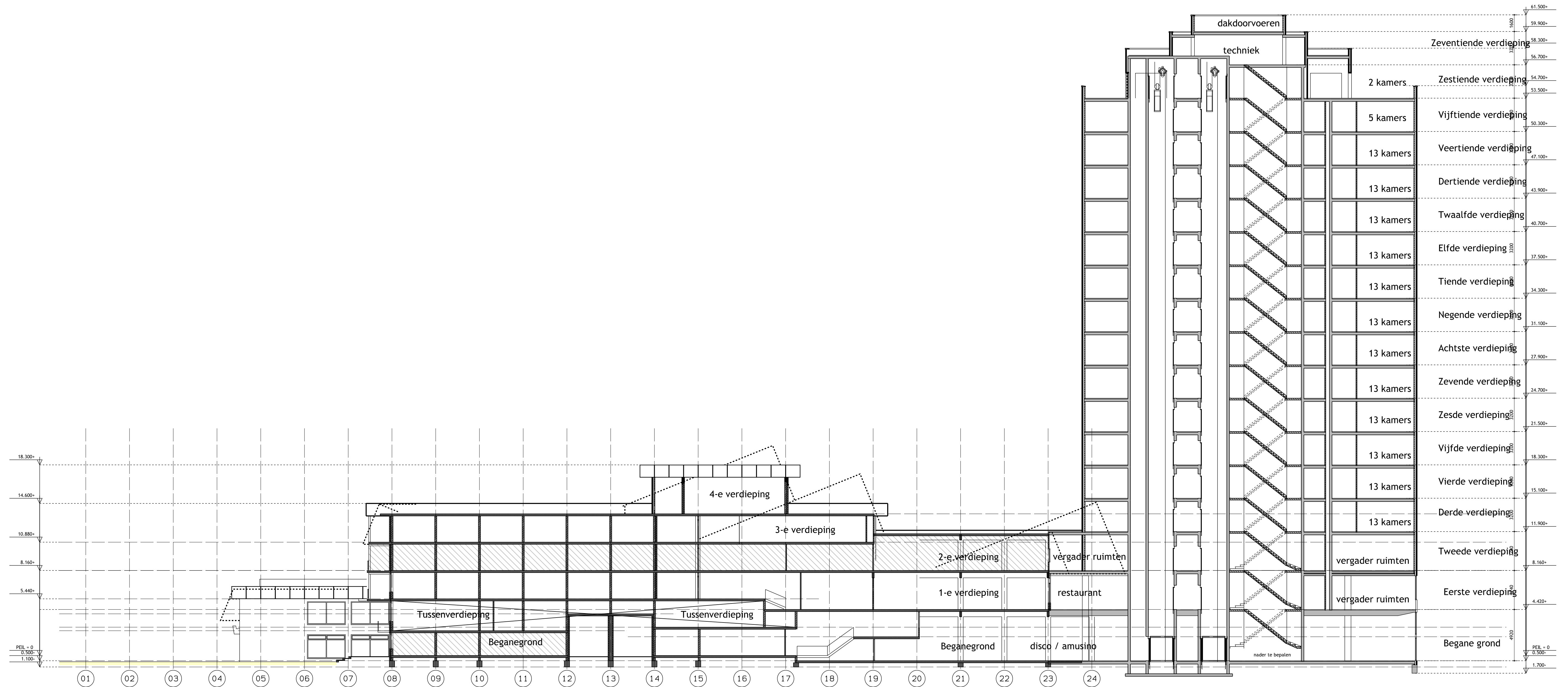
DOORSNEDE "BESTAAND"
