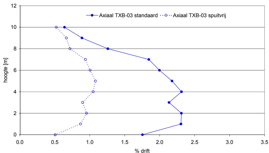
Figuur 5. Drift naar de lucht (% van de dosering) naast het perceel voor een standaard boomteeltspuit (axiaal uitgerust met TeeJet TXB 8003 spuitdoppen) en in combinatie met een 5 m spuitvrije zone in de volblad situatie (Stallinga et al. , 2009).
