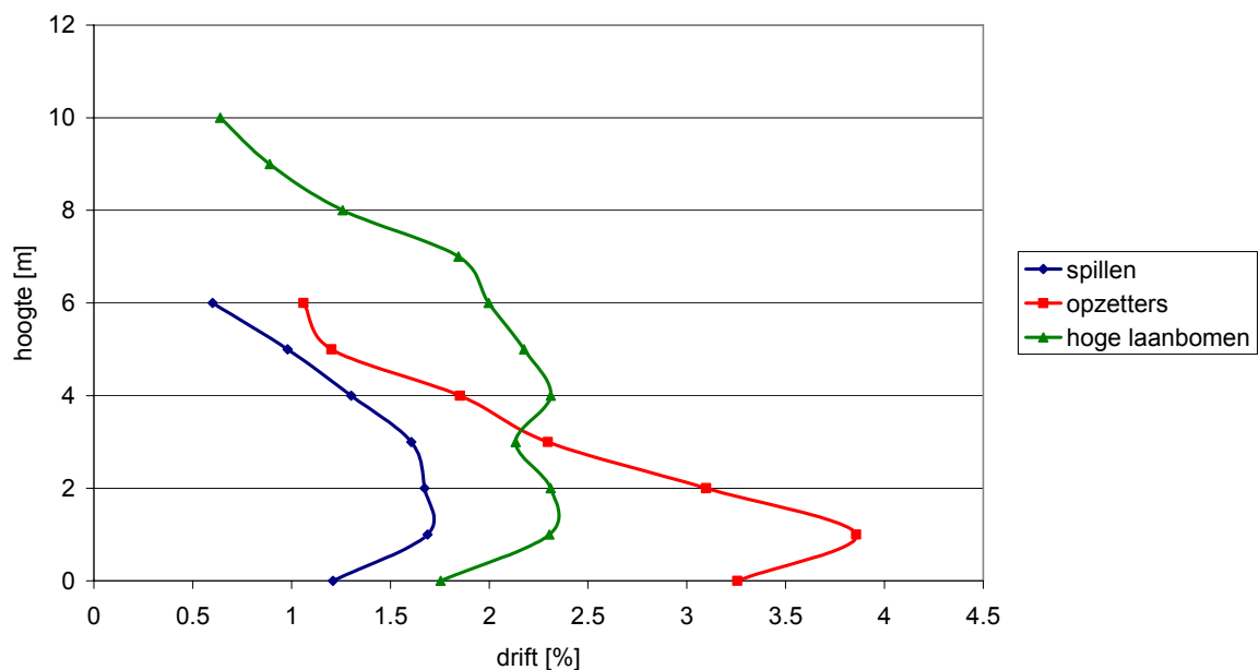
Figuur 3. Drift naar de lucht op 7,5 m afstand van de laatste bomenrij (% van de dosering) naast het perceel voor een standaard boomteeltspuit in de laanbomenteelt onderscheiden naar de boomvormen spil, opzetter en hoge laanboom
