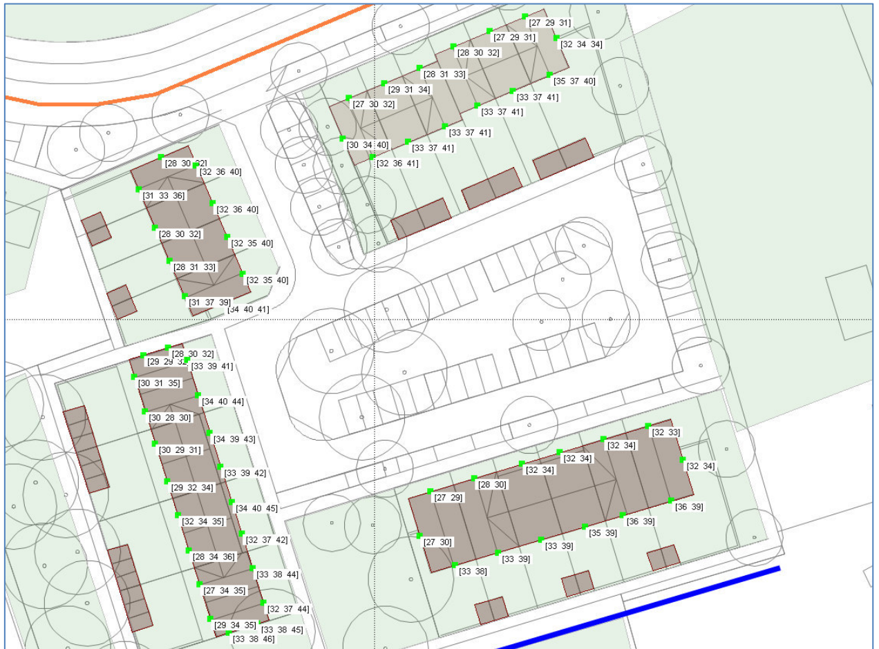
Figuur 10 Geluidbelasting ( L_{den} ) Van Geenstraat incl aftrek stiller verkeer
