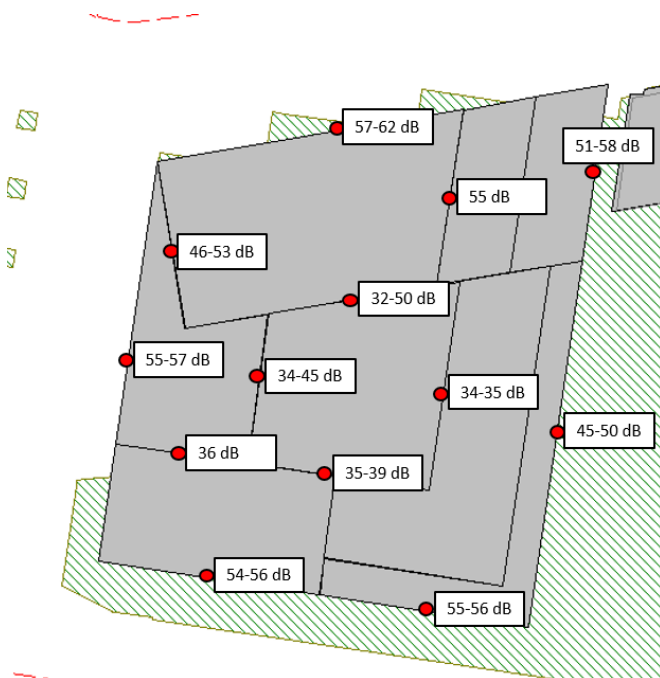
Figuur 9: Gecumuleerde geluidbelasting L_{den} (dB) ten gevolge van wegverkeer
