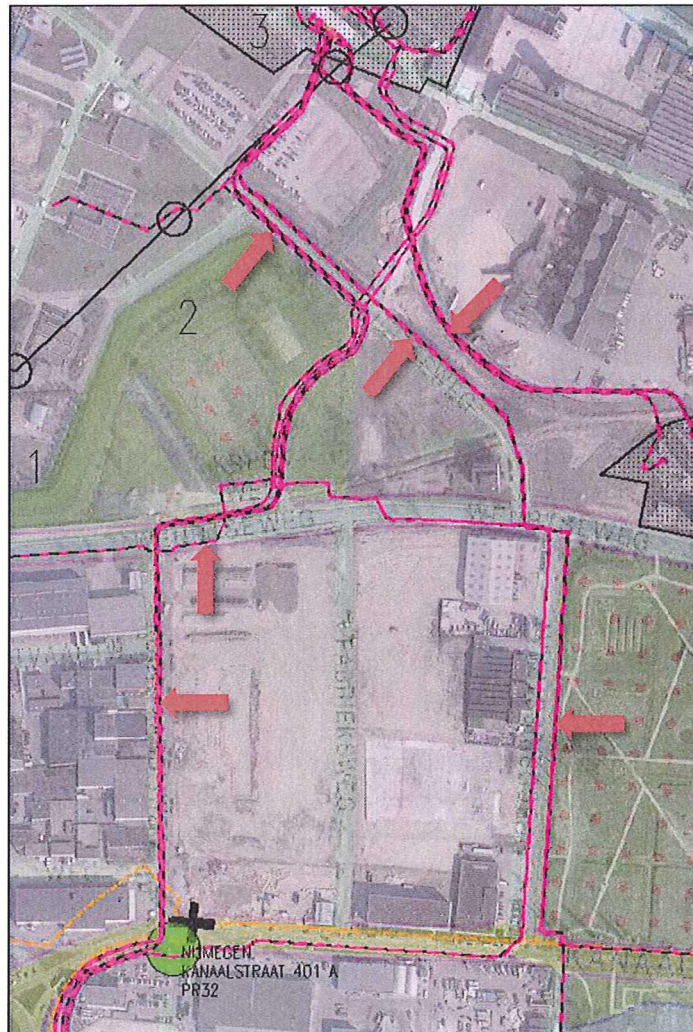
Afbeelding 1: ligging 50kV-kabelverbindingen
