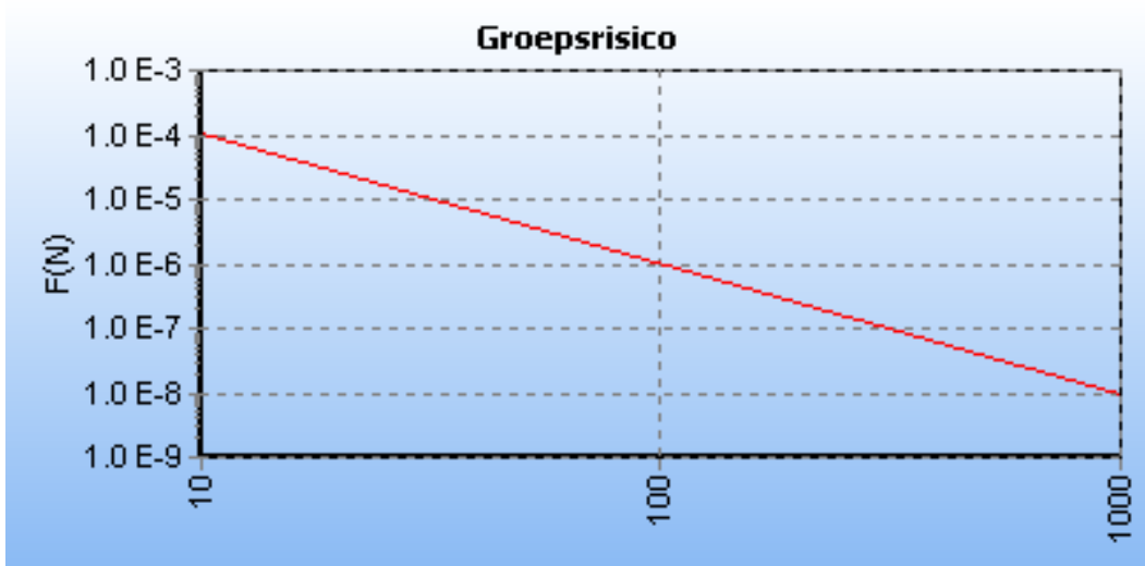
5.1 Figuur 5.1 FN curve voor N-578-04 van N.V. Nederlandse Gasunie voor de kilometer tussen stationing 11900.00 en stationing 12900.00
