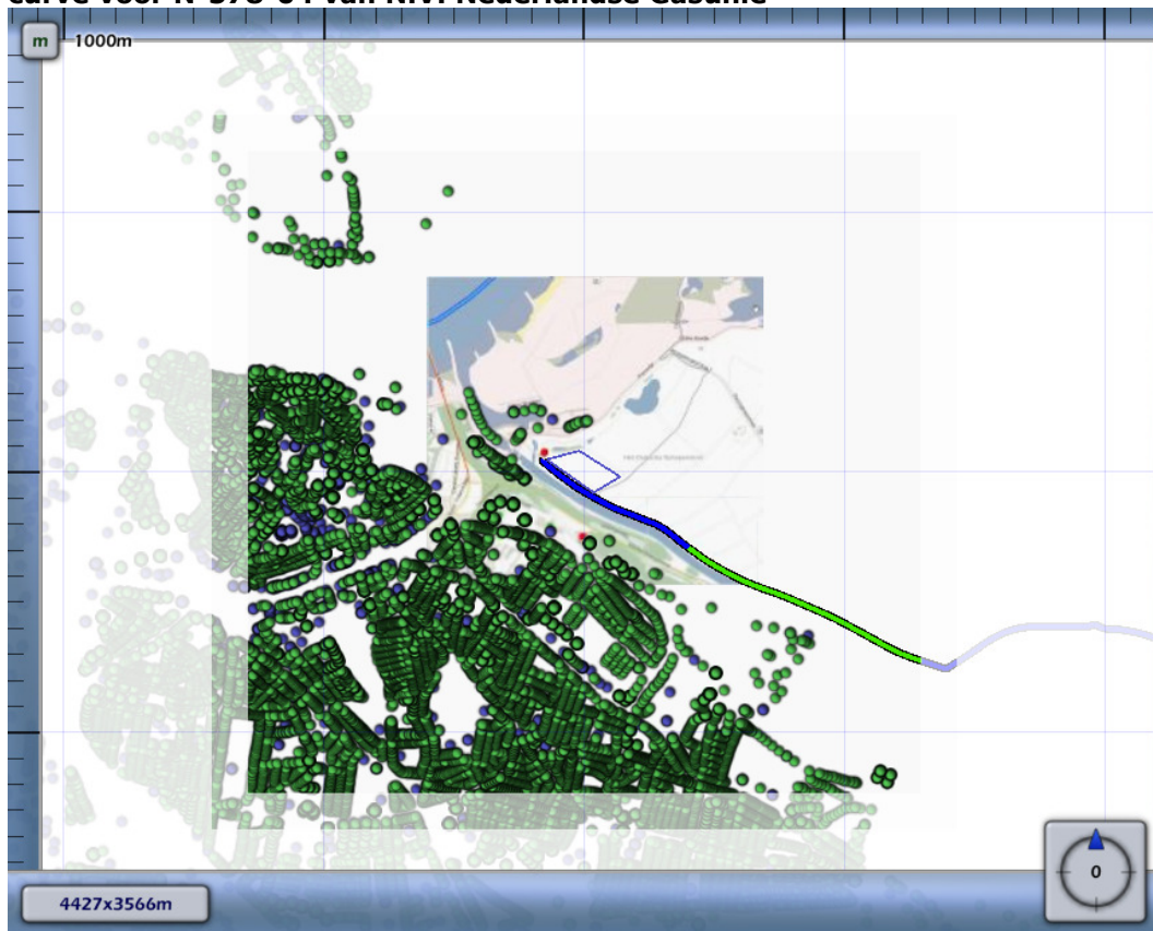
Figuur 4.1 Kilometer leiding behorende bij de maximale overschrijding van de FN-curve voor N-578-04 van N.V. Nederlandse Gasunie
