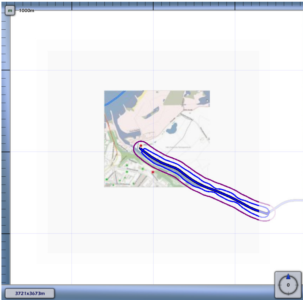
3.1 Figuur 3.1 Plaatsgebonden risico voor N-578-04 van N.V. Nederlandse Gasunie
