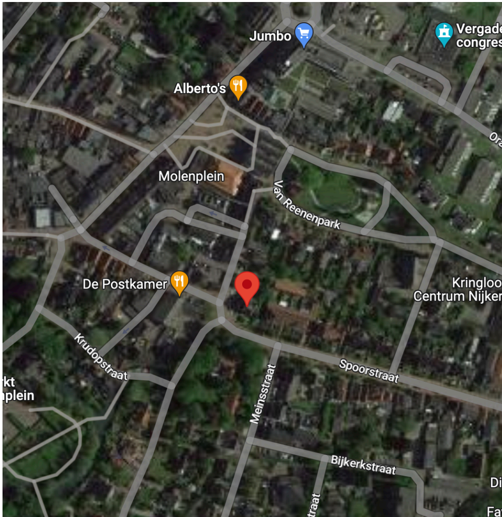
Afb. 1: Kaart plangebied
