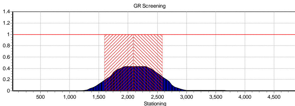
Figuur 5 Overschrijdingsfactor uitgezet tegen stationing van de A-510-KR-063-1 t/m 069, zonder extra dekking, bestaande situatie. Het rood gearceerde deel geeft de kilometer aan waarover de FN-curve is berekend.
