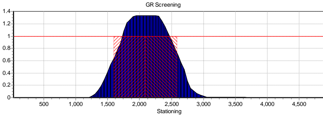
Figuur 3 Overschrijdingsfactor uitgezet tegen stationing van de A-510-KR-063-1 t/m 069, zonder extra dekking, situatie met bouwplannen Fase 1 t/m 4. Het rood gearceerde deel geeft de kilometer aan waarover de FN-curve is berekend.
