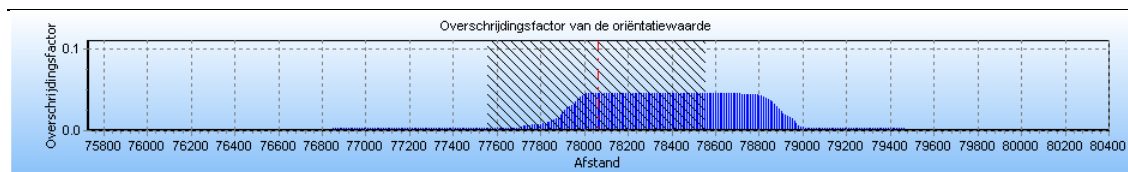
Figuur 4.5 Groepsrisicoscreening voor leiding A-510 van de Nederlandse Gasunie, situatie 2
