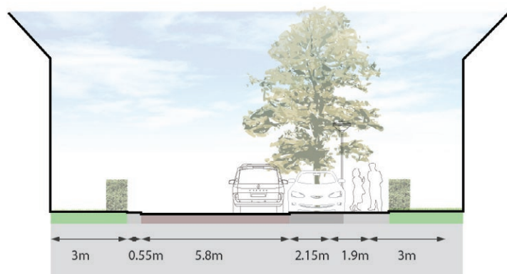
Principeprofiel ontsluiting
