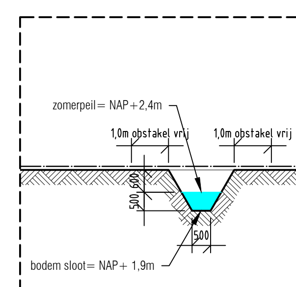
DETAIL SLOOT T.P.V. LAARSTRAAT
