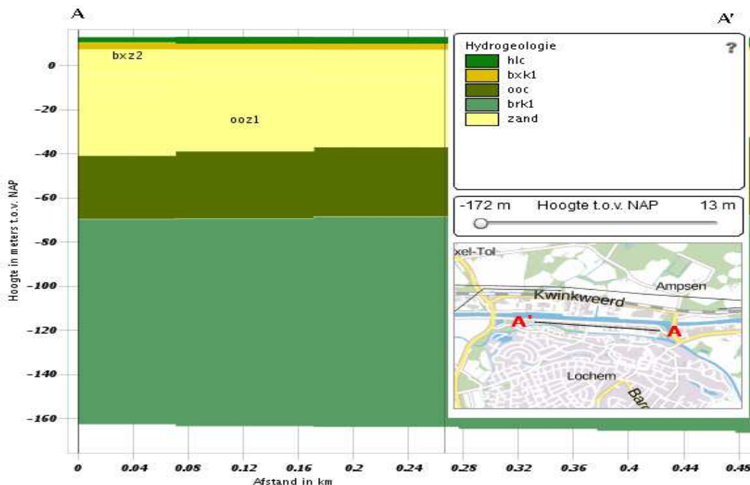
Figuur 3.2 Verticale dwarsdoorsnede van het plangebied
