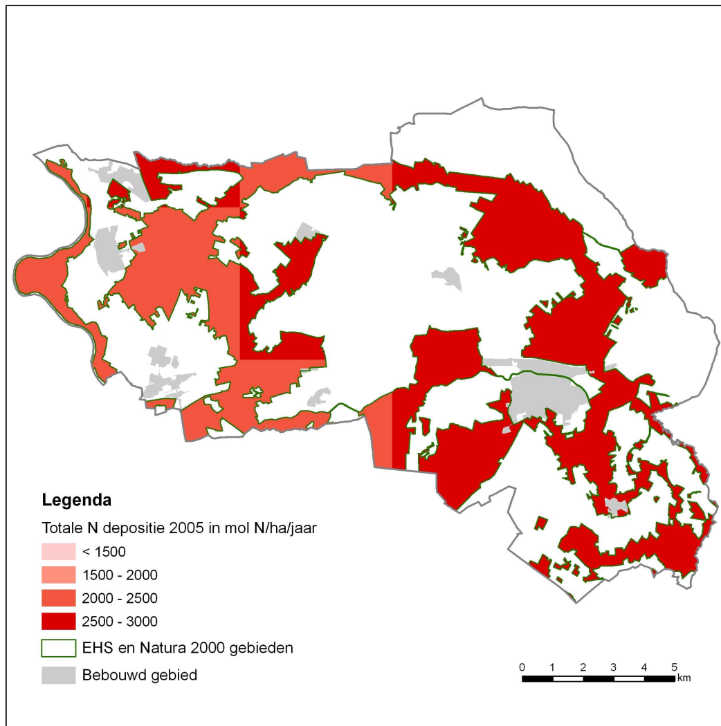
Figuur 3 Totale atmosferische N-depositie (mol N ha -1 jr -1 ) op de EHS- en Natura 2000-gebieden in 2005.
