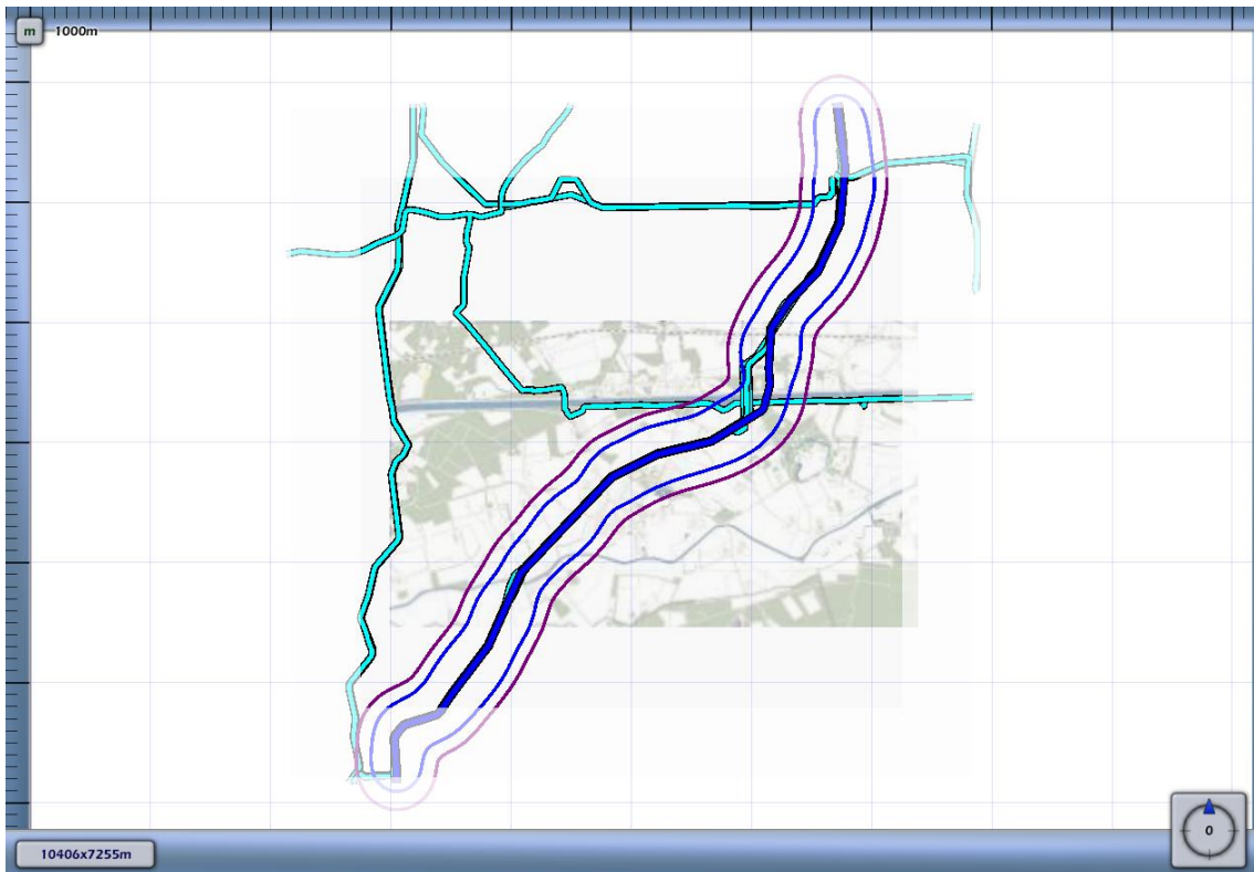
3.1 Figuur 3.2 Plaatsgebonden risico voor A-505 van N.V. Nederlandse Gasunie
