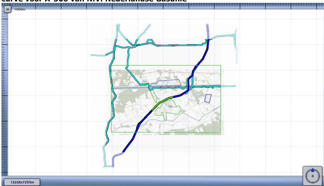
Figuur 4.3 Kilometer leiding behorende bij de maximale overschrijding van de FN-curve voor A-506 van N.V. Nederlandse Gasunie
