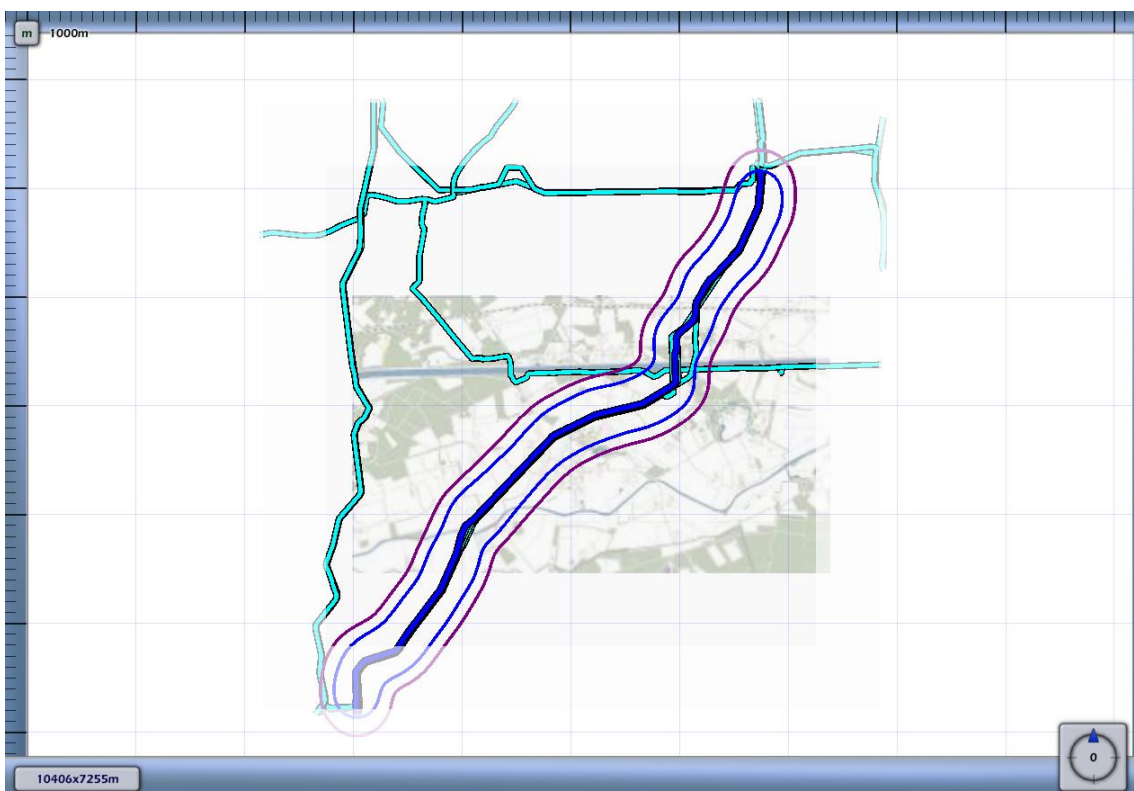
3.3 Figuur 3.12 Plaatsgebonden risico voor A-608 van N.V. Nederlandse Gasunie
