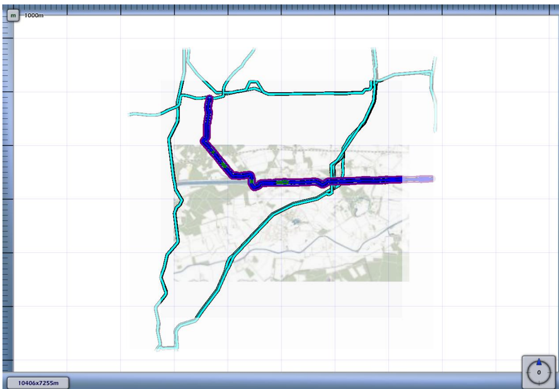
3.5 Figuur 3.19 Plaatsgebonden risico voor N-560-07 van N.V. Nederlandse Gasunie
