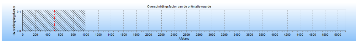
4.5 Figuur 4.19 Groepsrisico screening voor N-560-07 van N.V. Nederlandse Gasunie
