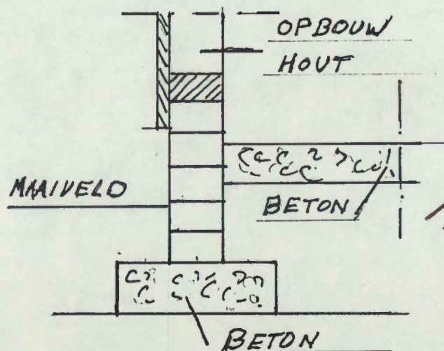
DOORSNEDE
