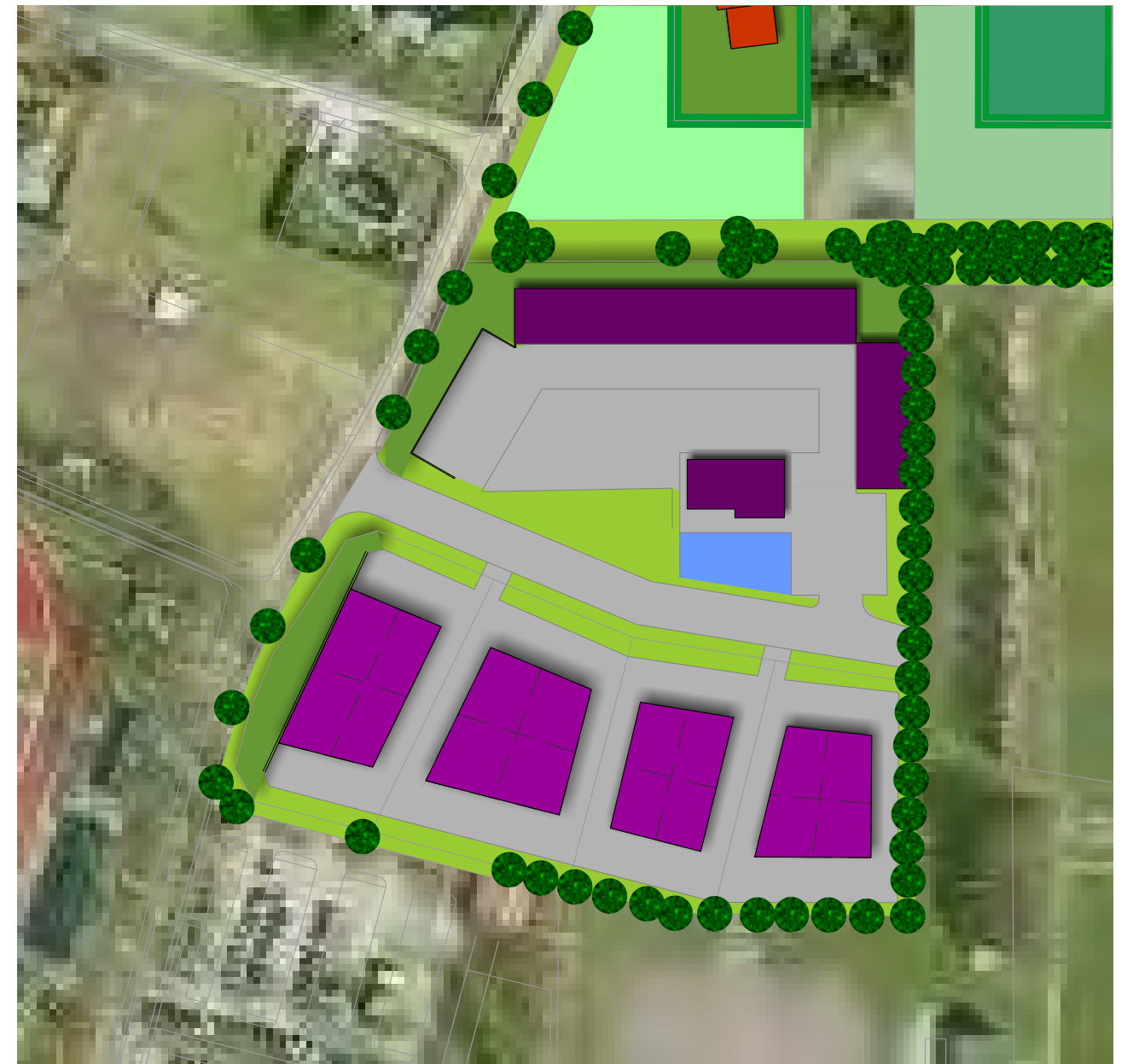
afbeelding 42: Detail stedenbouwkundig ontwerp
