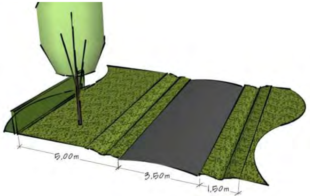
afbeelding 52: Doorsnede Eeuwlandseweg
