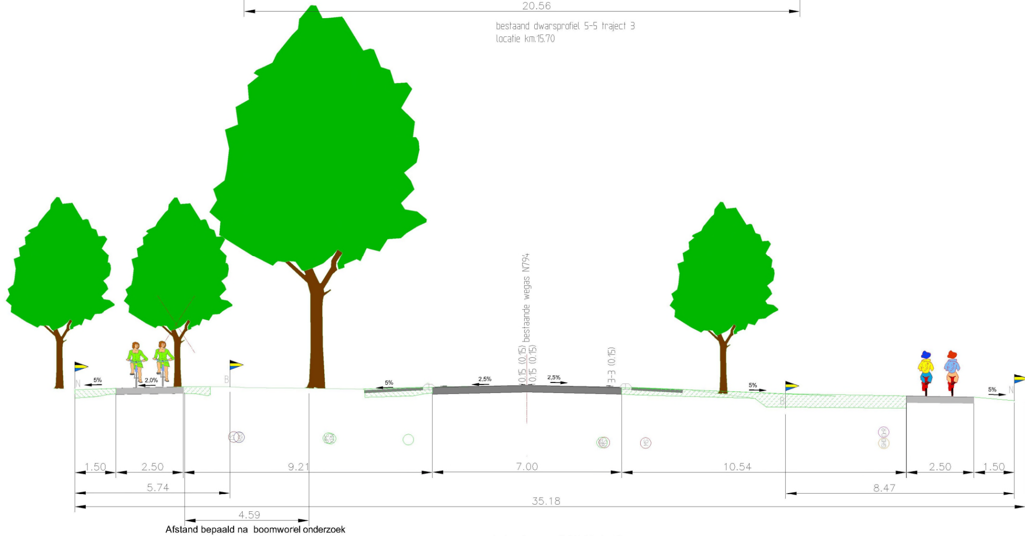
principe dwarsprofiel 5-5 traject 3 locatie km.15.70
