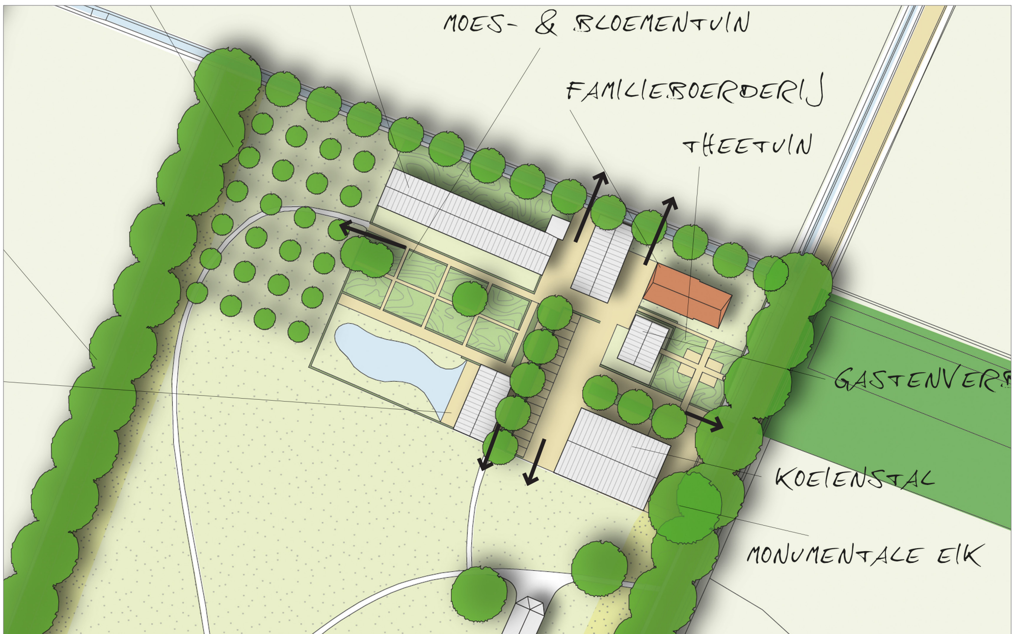
Uitsnede erf
