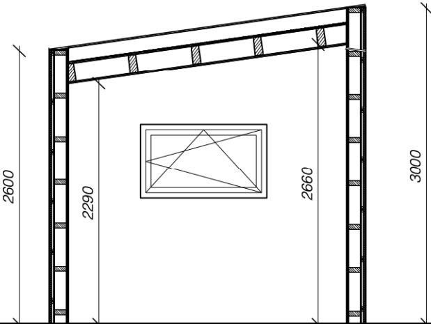
doorsnede
