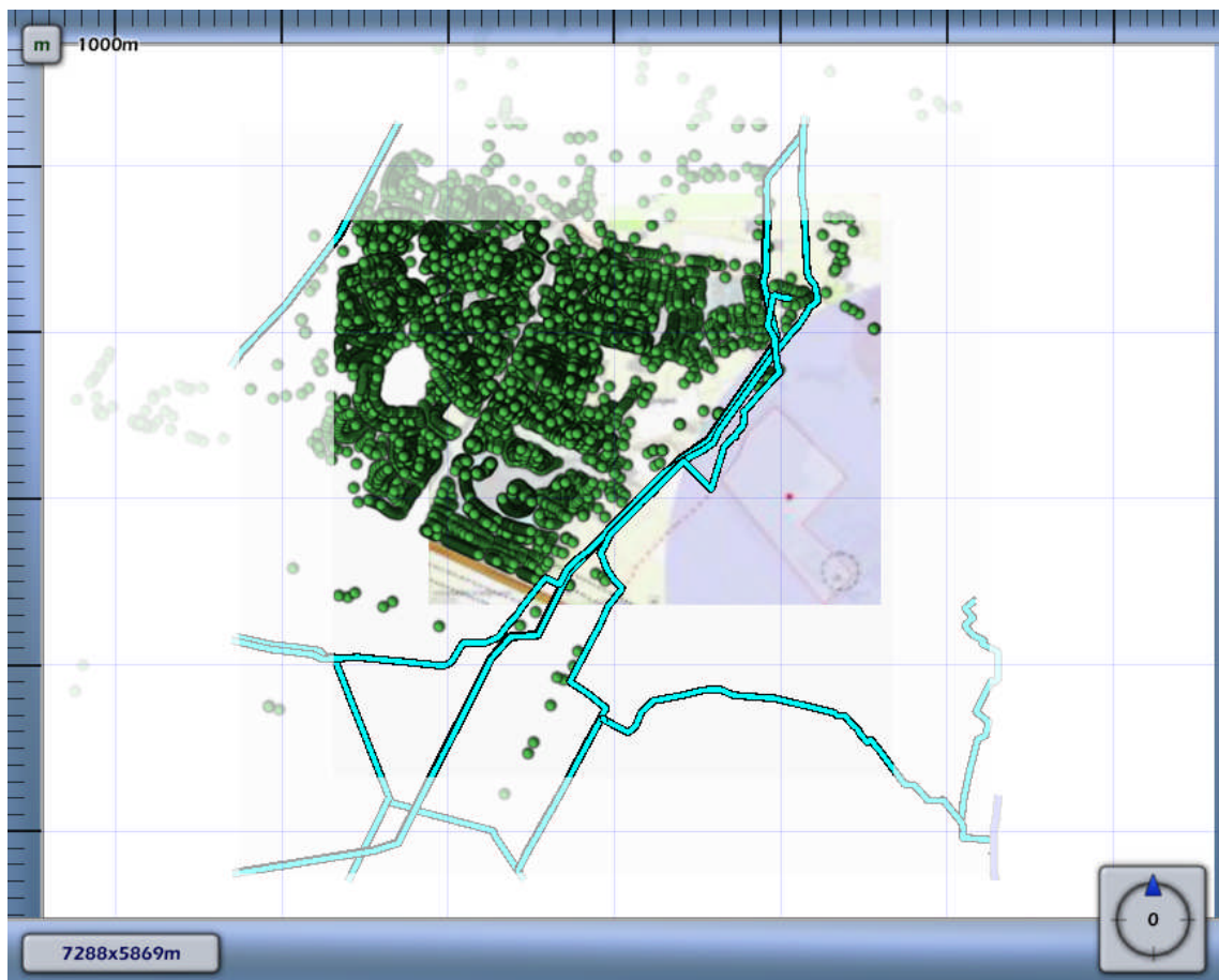
4.10 Figuur 4.10 Groepsrisico screening voor N-576-68 van N.V. Nederlandse Gasunie
