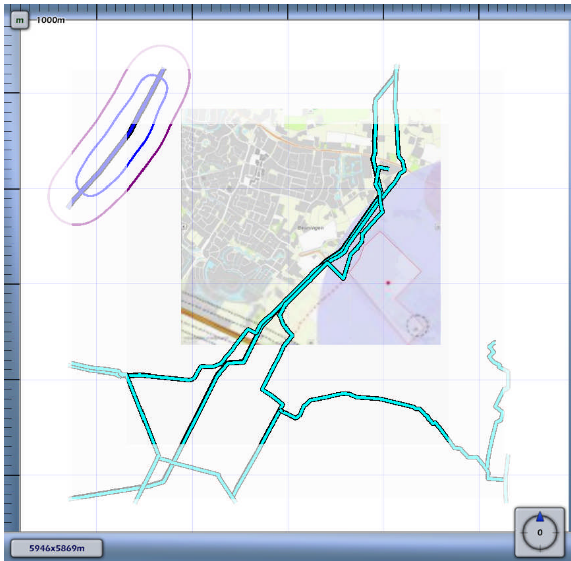
3.2 Figuur 3.2 Plaatsgebonden risico voor A-507 van N.V. Nederlandse Gasunie
