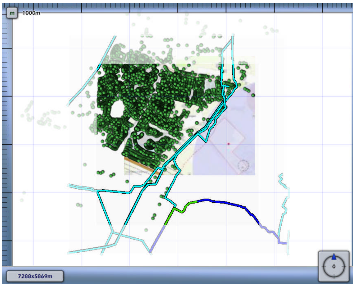
4.8 Figuur 4.8 Groepsrisico screening voor N-576-04 van N.V. Nederlandse Gasunie
