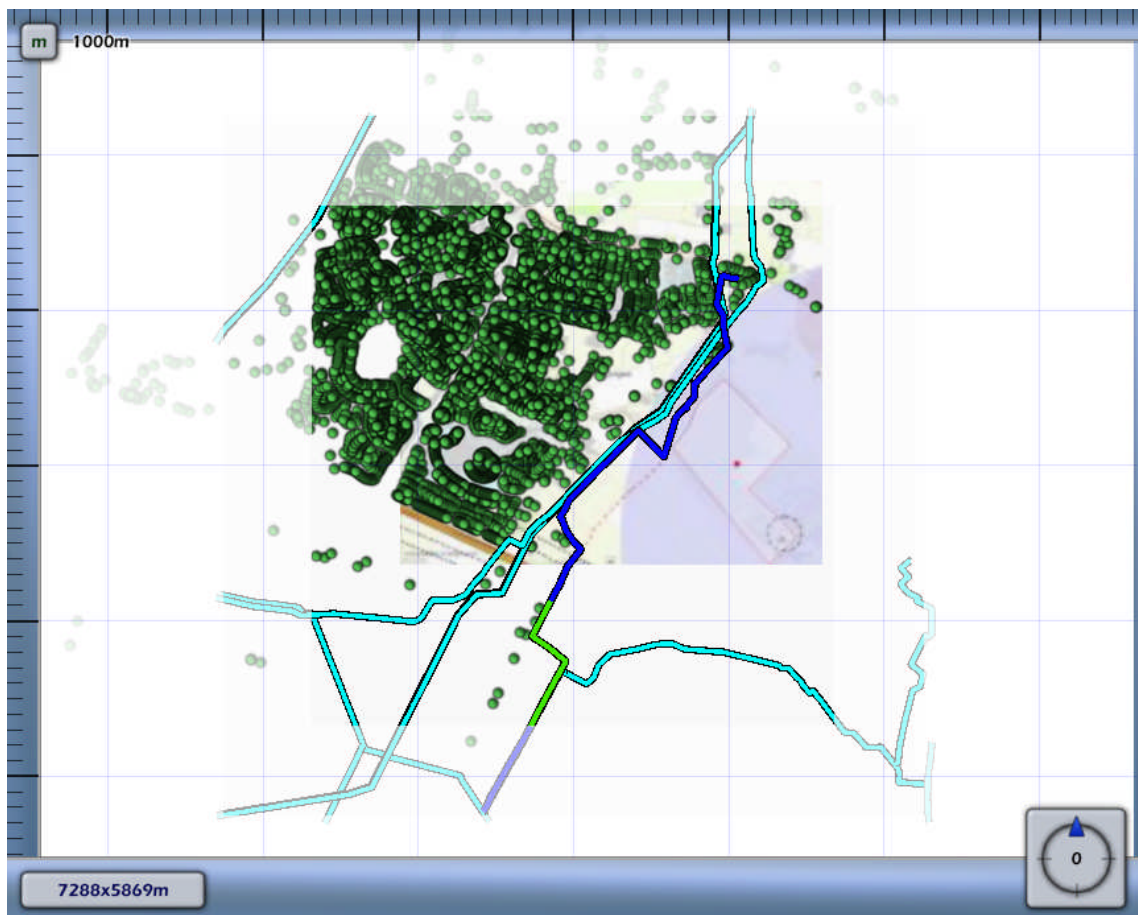
4.7 Figuur 4.7 Groepsrisico screening voor N-576-02 van N.V. Nederlandse Gasunie
