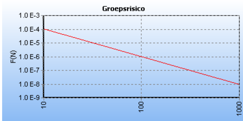
5.7 Figuur 5.7 FN curve voor N-576-02 van N.V. Nederlandse Gasunie voor de kilometer tussen stationing 640.00 en stationing 1640.00
