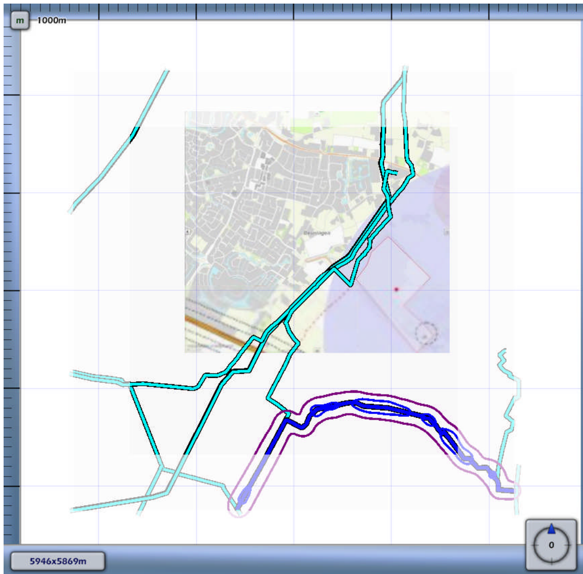
3.7 Figuur 3.7 Plaatsgebonden risico voor N-576-02 van N.V. Nederlandse Gasunie
