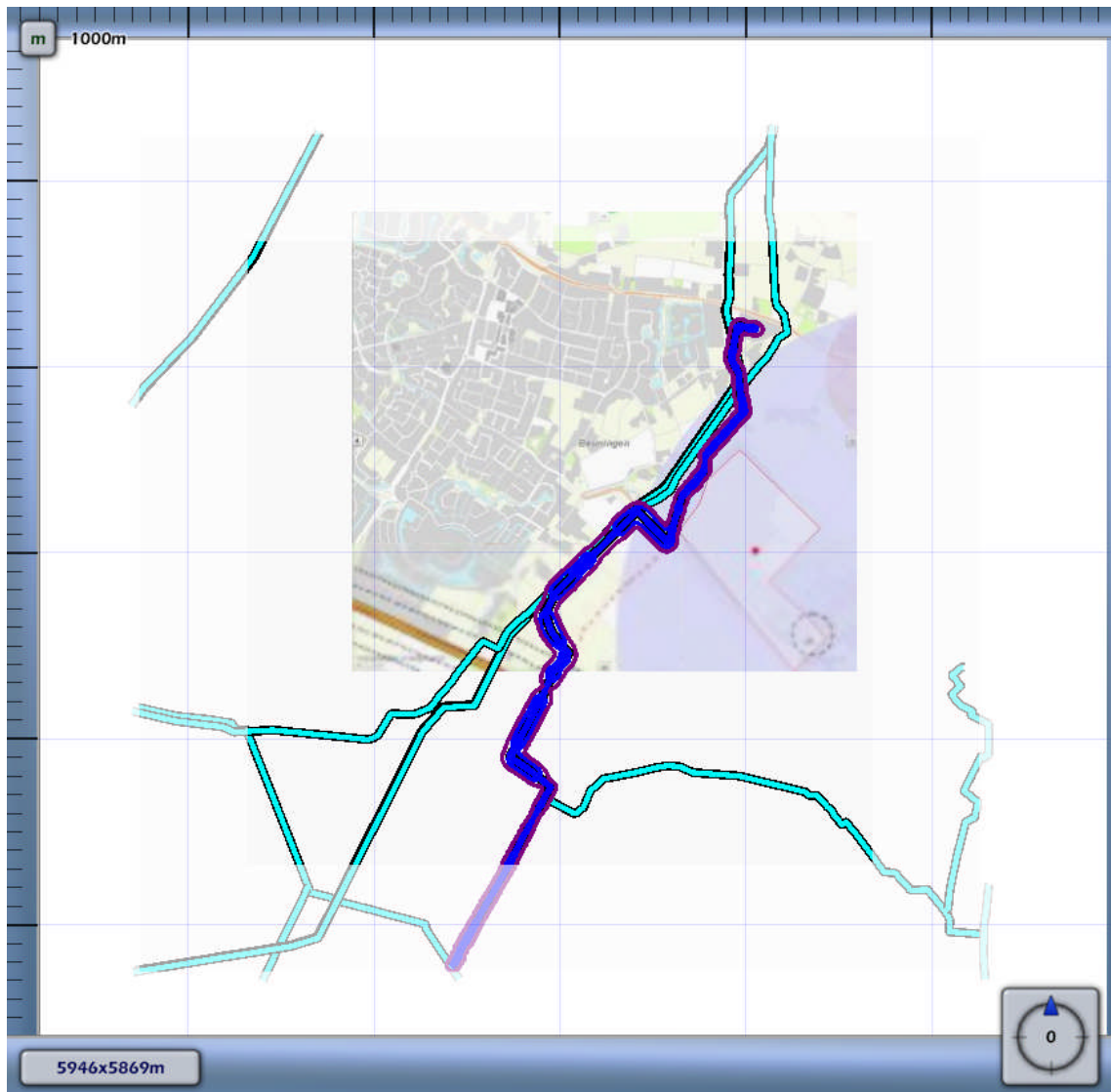
3.6 Figuur 3.6 Plaatsgebonden risico voor N-576-01 van N.V. Nederlandse Gasunie
