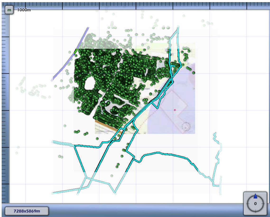
4.2 Figuur 4.2 Groepsrisico screening voor A-507 van N.V. Nederlandse Gasunie
