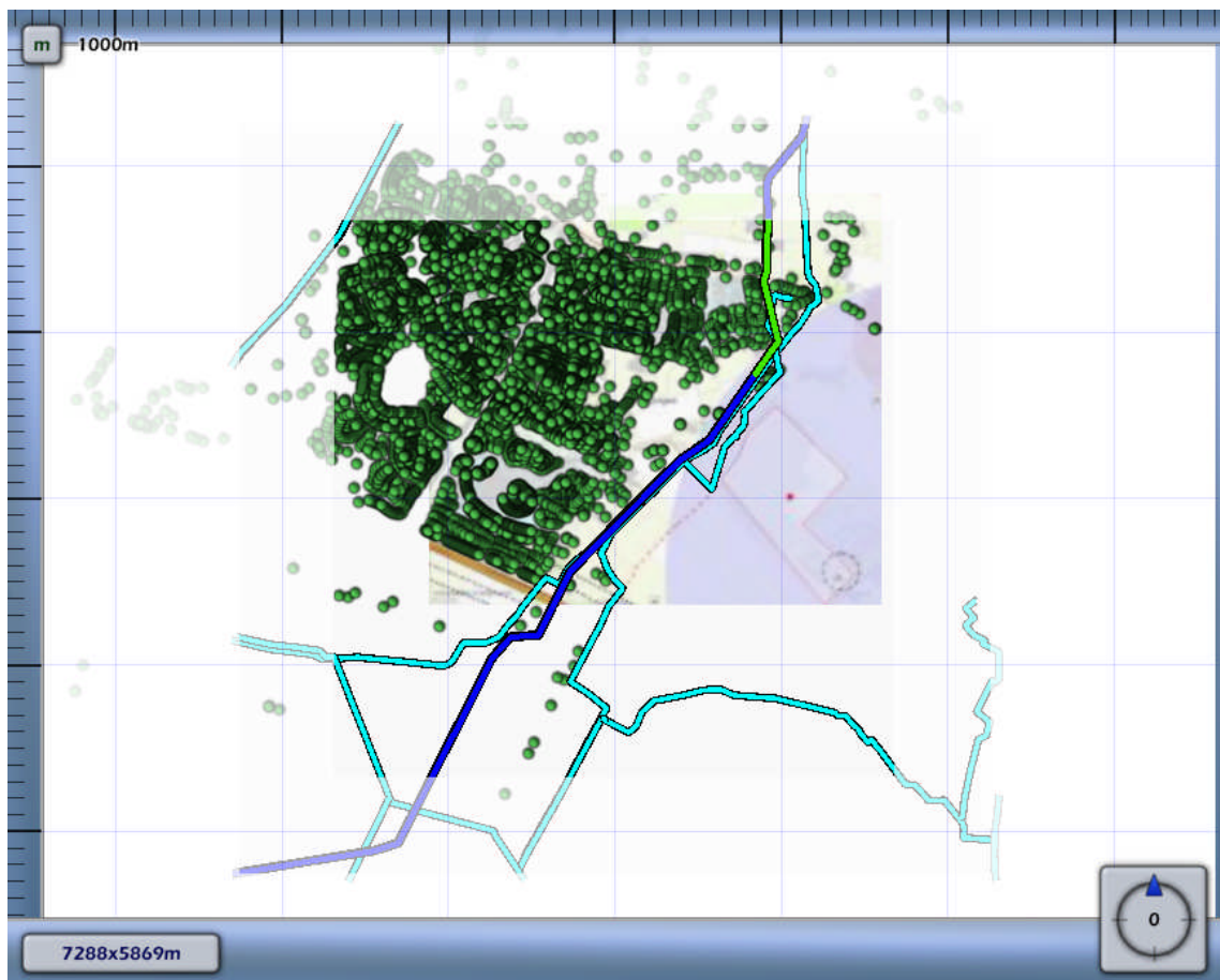
4.5 Figuur 4.5 Groepsrisico screening voor A-663 van N.V. Nederlandse Gasunie
