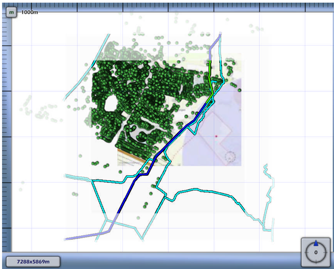
4.4 Figuur 4.4 Groepsrisico screening voor A-533 van N.V. Nederlandse Gasunie
