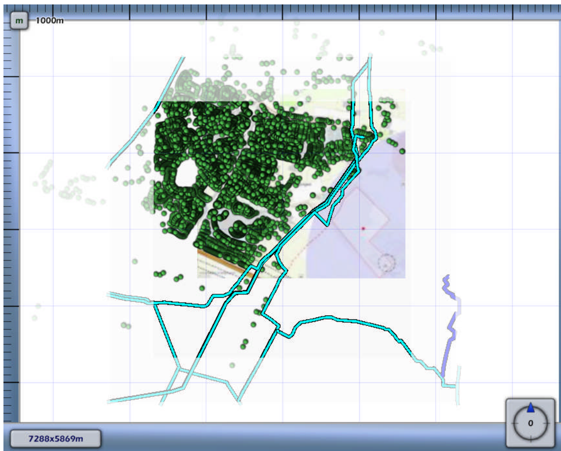
4.11 Figuur 4.11 Groepsrisico screening voor N-576-70 van N.V. Nederlandse Gasunie
