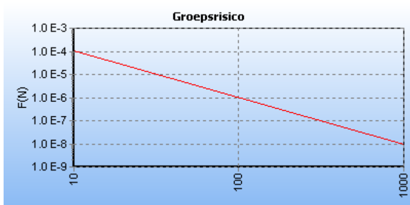
5.11 Figuur 5.11 FN curve voor N-576-70 van N.V. Nederlandse Gasunie voor de kilometer tussen stationing 2030.00 en stationing 2800.00
