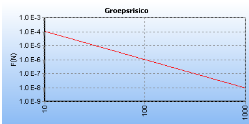
5.8 Figuur 5.8 FN curve voor N-576-04 van N.V. Nederlandse Gasunie voor de kilometer tussen stationing 0.00 en stationing 20.00
