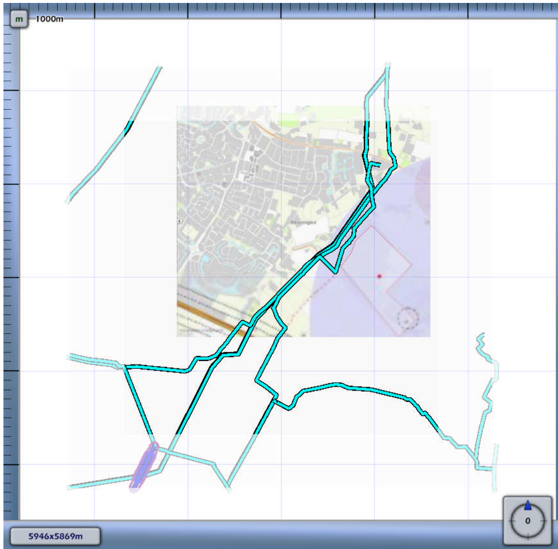
3.12 Figuur 3.12 Plaatsgebonden risico voor N-576-71 van N.V. Nederlandse Gasunie
