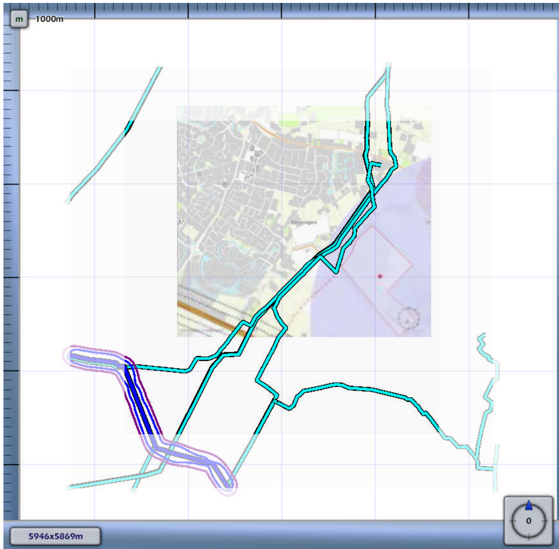
3.11 Figuur 3.11 Plaatsgebonden risico voor N-576-70 van N.V. Nederlandse Gasunie
