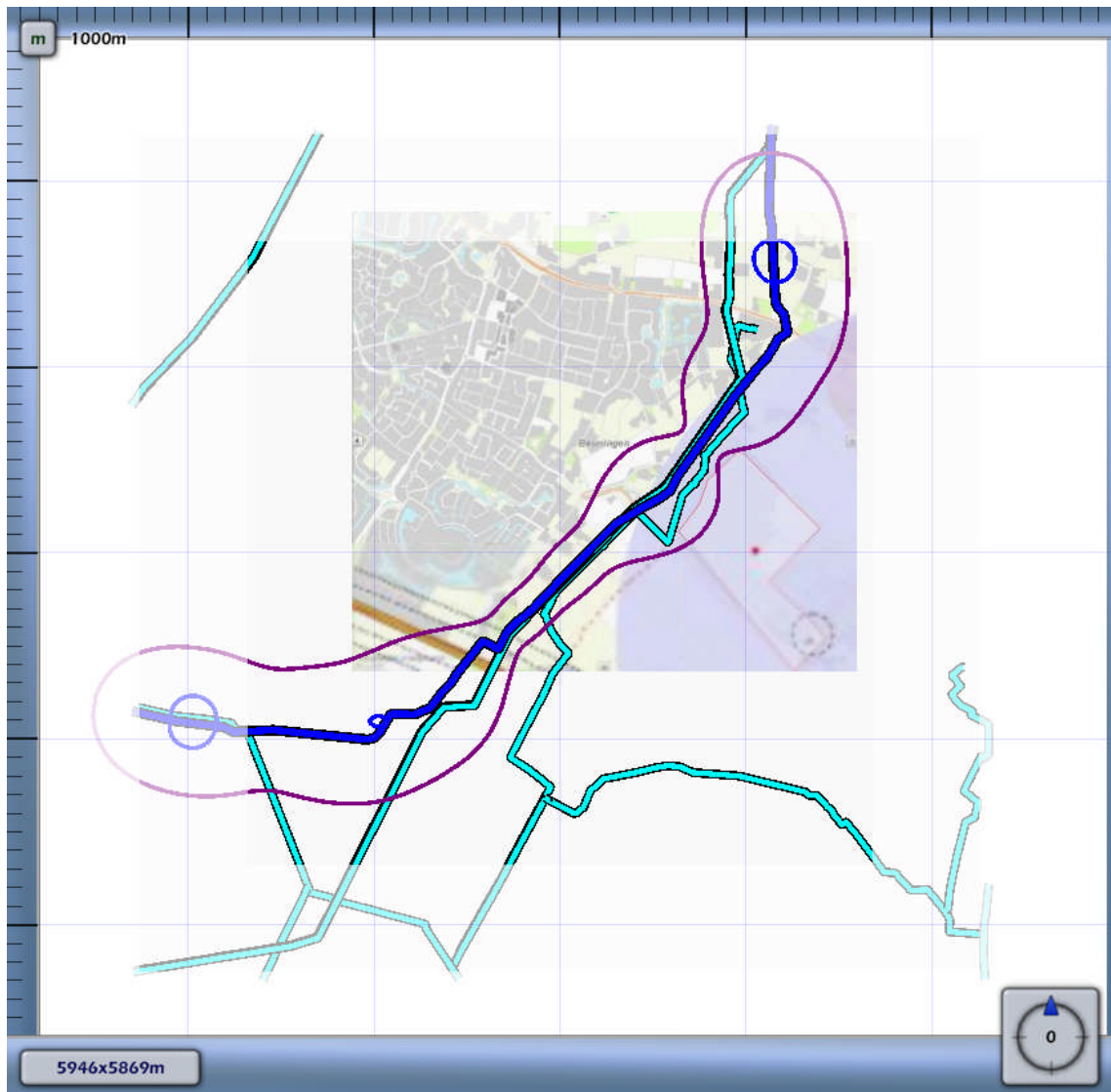
3.5 Figuur 3.5 Plaatsgebonden risico voor A-663 van N.V. Nederlandse Gasunie
