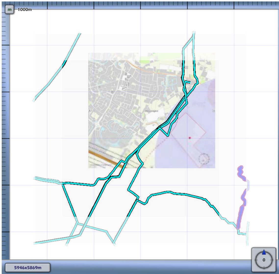
3.10 Figuur 3.10 Plaatsgebonden risico voor N-576-68 van N.V. Nederlandse Gasunie
