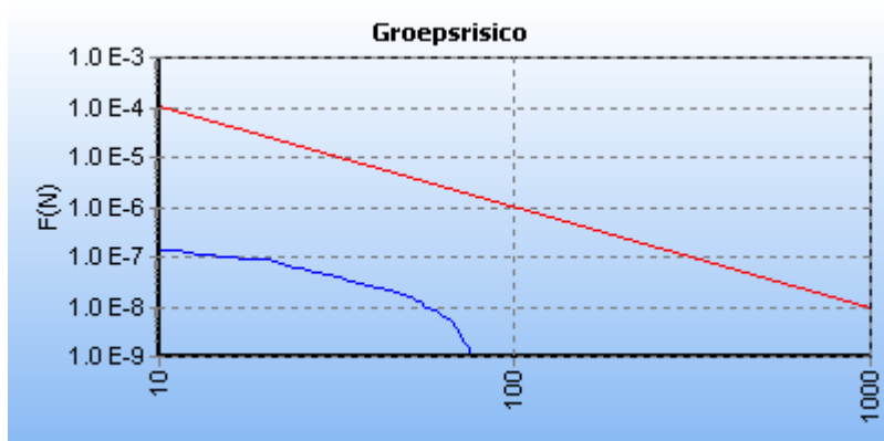
5.5 Figuur 5.5 FN curve voor A-663 van N.V. Nederlandse Gasunie voor de kilometer tussen stationing 29410.00 en stationing 30410.00
