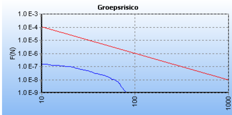
5.4 Figuur 5.4 FN curve voor A-533 van N.V. Nederlandse Gasunie voor de kilometer tussen stationing 27590.00 en stationing 28590.00
