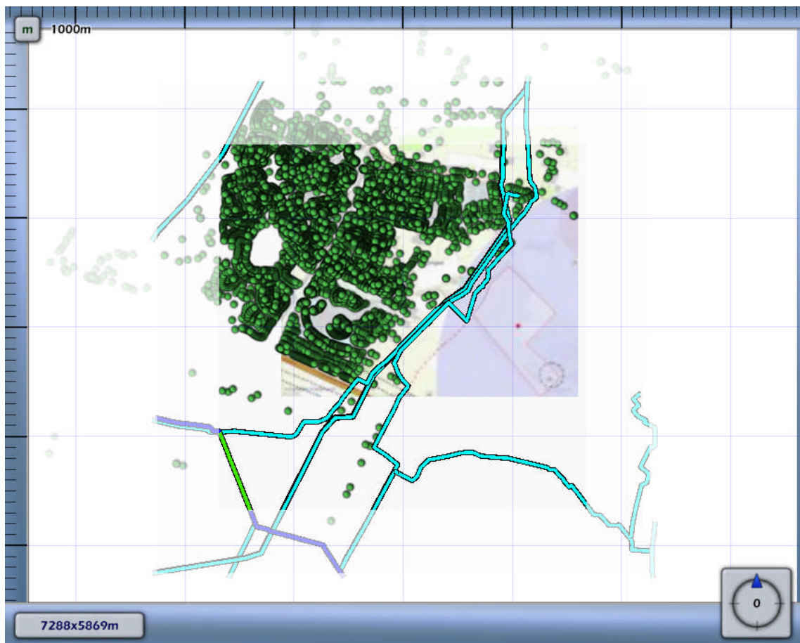
4.12 Figuur 4.12 Groepsrisico screening voor N-576-71 van N.V. Nederlandse Gasunie
