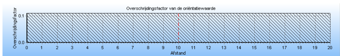
4.8 Figuur 4.8 Groepsrisico screening voor N-576-04 van N.V. Nederlandse Gasunie
