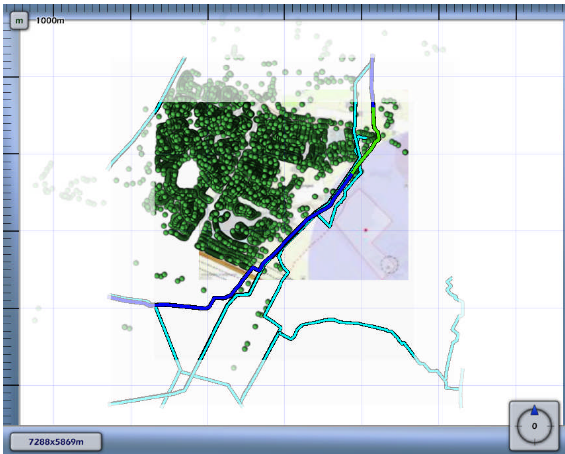
4.6 Figuur 4.6 Groepsrisico screening voor N-576-01 van N.V. Nederlandse Gasunie
