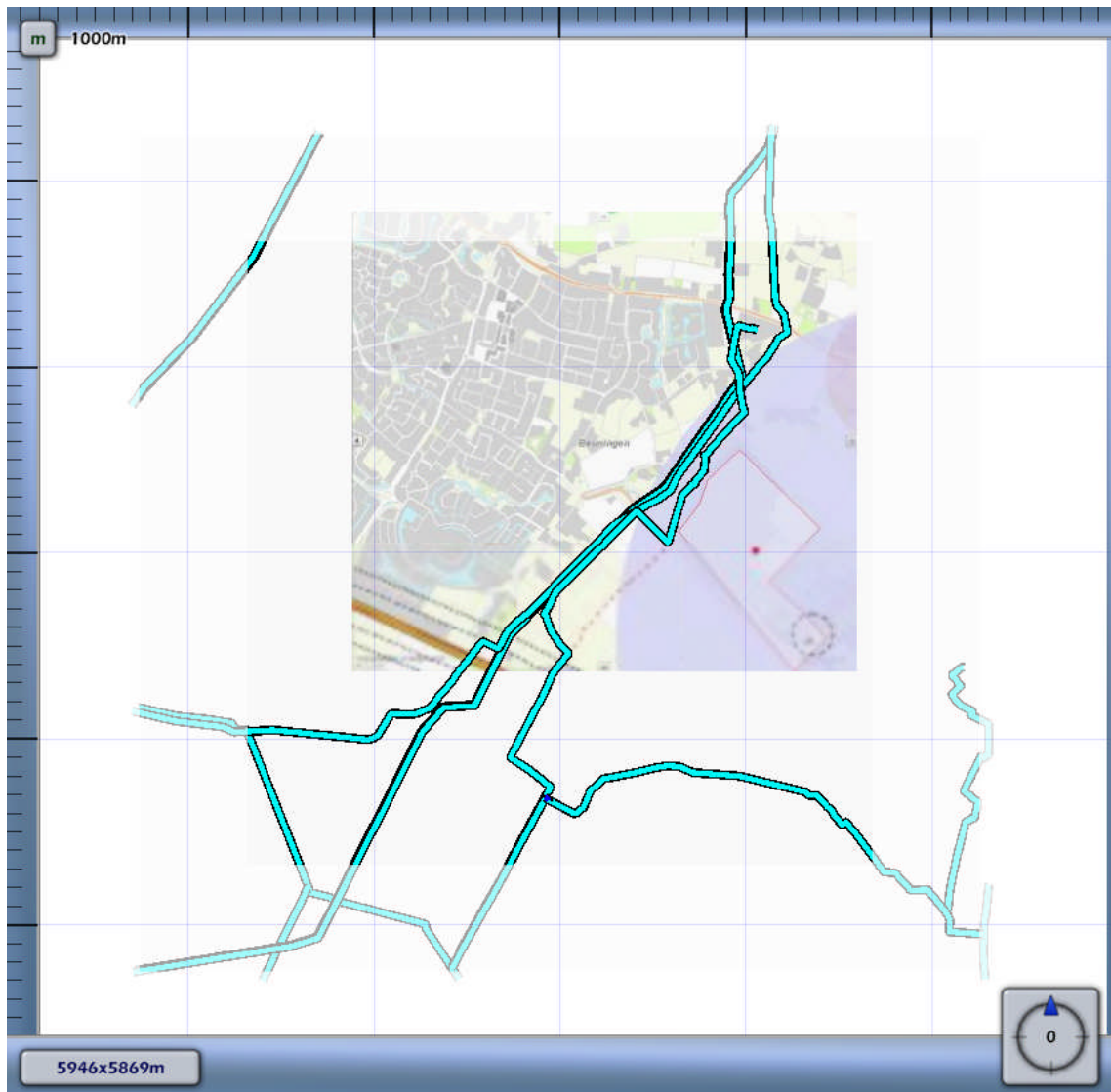
3.8 Figuur 3.8 Plaatsgebonden risico voor N-576-04 van N.V. Nederlandse Gasunie
