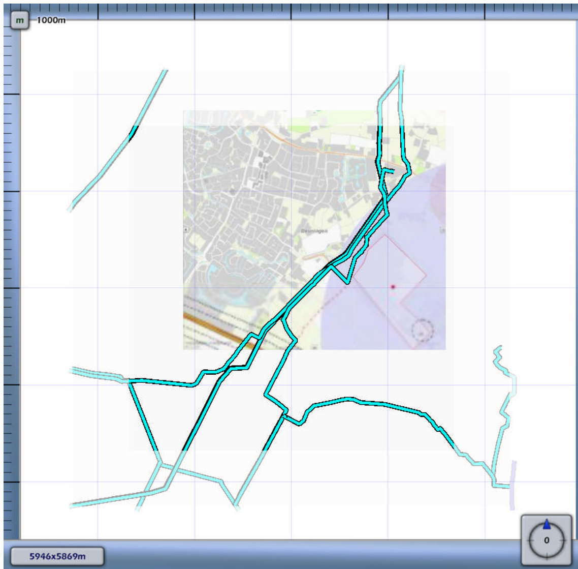
3.9 Figuur 3.9 Plaatsgebonden risico voor N-576-67 van N.V. Nederlandse Gasunie
