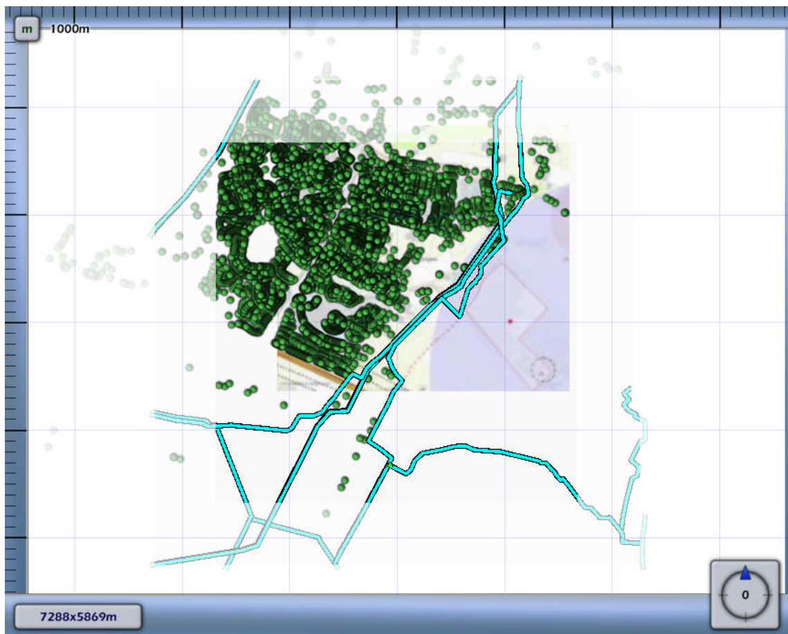
4.9 Figuur 4.9 Groepsrisico screening voor N-576-67 van N.V. Nederlandse Gasunie
