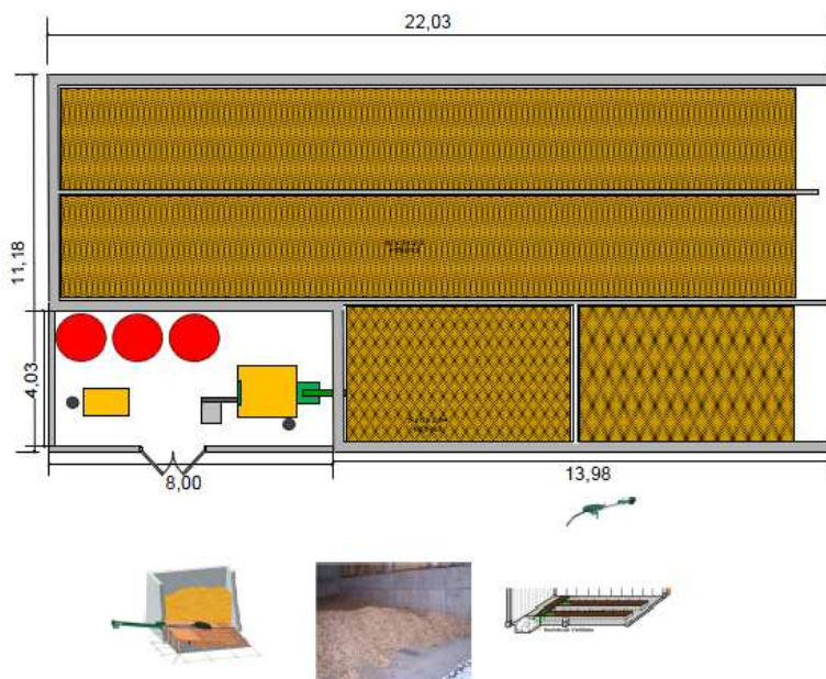
Figuur: indeling bijgebouw biomassa
