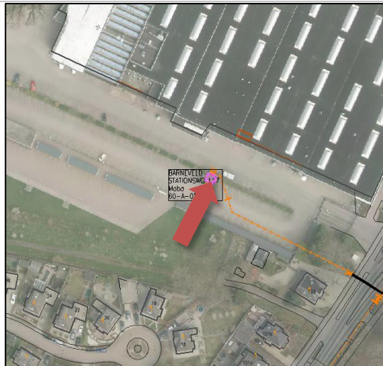
Afbeelding 4b: Ligging gasdrukmeet- en regelstation (rode pijl).
