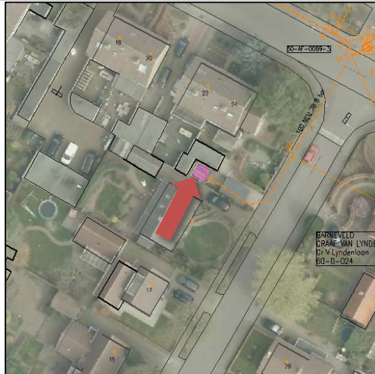
Afbeelding 2b: Ligging gasdrukmeet- en regelstation (rode pijl).
