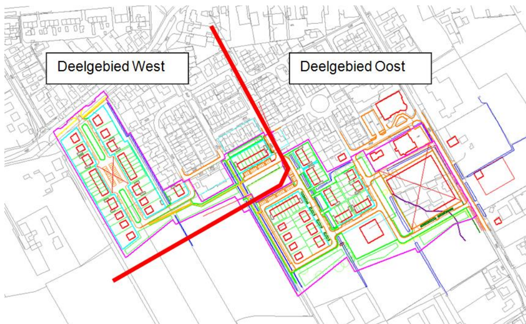
Figuur 9: Deelgebieden t.b.v. waterberging en afvoer
