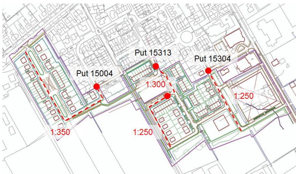
Figuur 11: Aansluitlocaties afvalwaterriolering, langste tracés en afschotten
