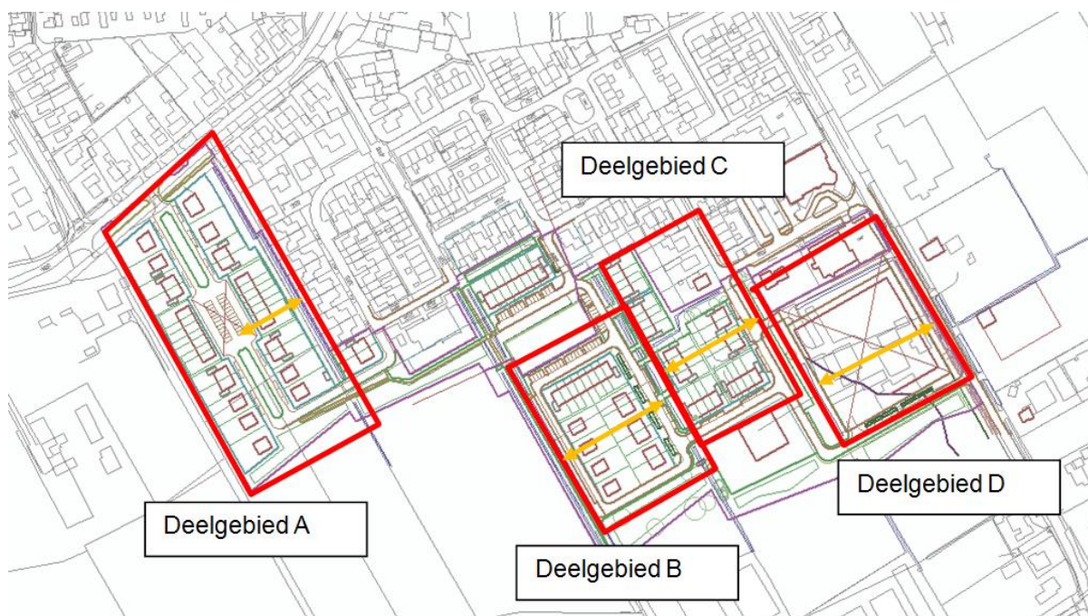
Figuur 13: Deelgebieden t.b.v. berekening van de ontwatering (oranje peil: berekening maatgevende opbolling)
