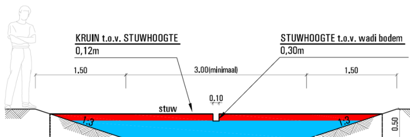
Figuur 10: Doorsnede wadi en stuw
